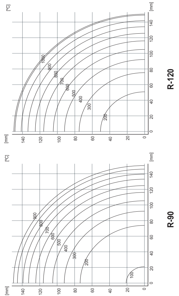
Figura A.6.7.4.e. Isotermas de un cuarto de sección circular de 300 mm de diámetro expuesta perimetralmente
