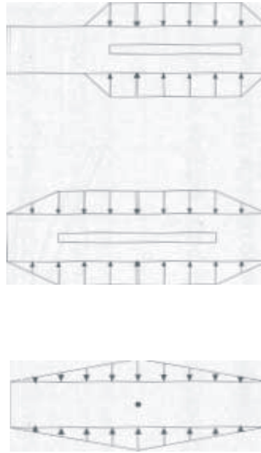
Figura A.12.5.2.4.c. Factores de distribución de carga para cargas puntuales en el borde ( b=1,20\text{ m} )
