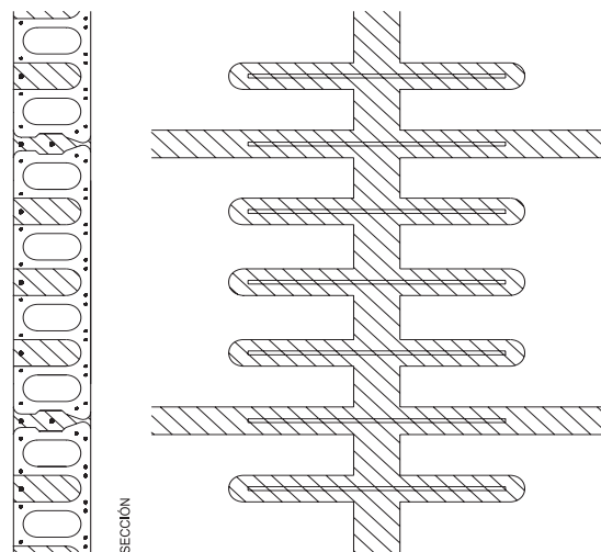
Figura 59.2.4.a Armadura superior en losas alveolares pretensadas
