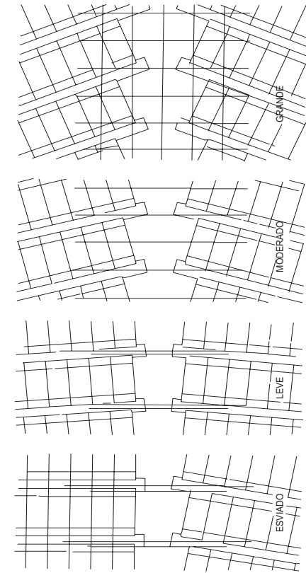
Figura A.12.8.1.c Encuentro oblicuo de viguetas
