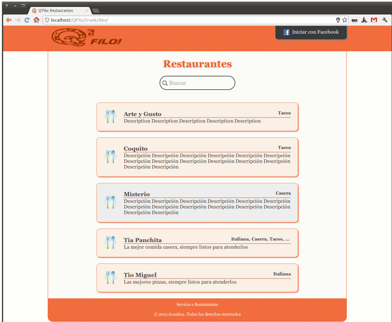
Figura 3: Página inicial.
