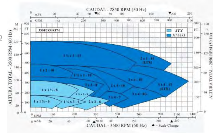
BOMBA MARCA DELTA-SIVAN MODELO D196 TAMAÑO MTX/LTX.
