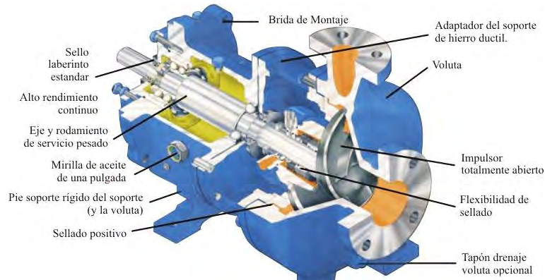
BOMBA MARCA DELTA-SIVAN MODELO D196 TAMAÑO STX.
