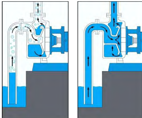
CEBADO DE BOMBA MARCA DELTA-SIVAN MODELO D796 MTX.
