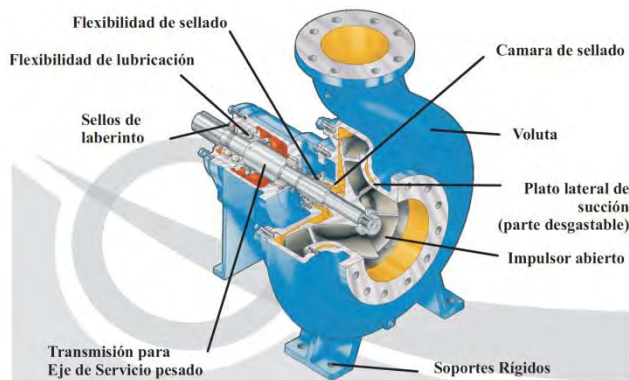
BOMBA MARCA DELTA-SIVAN MODELO D180 TAMAÑO L.
