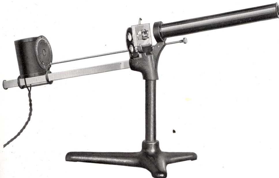
M615A Axometer
