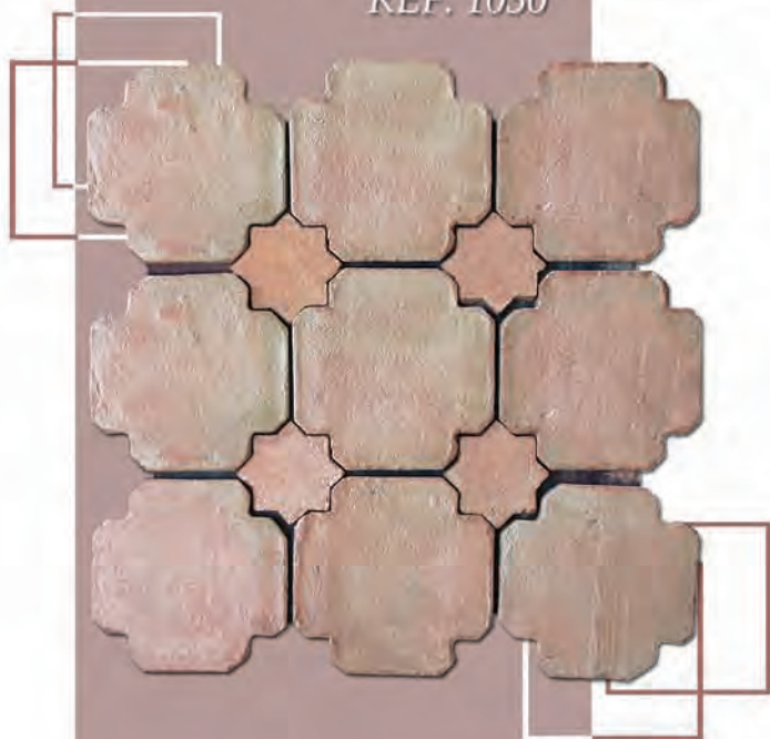
Losa de 24 x 24 cm. combinada con Estrella de 10 x 10 cm.
