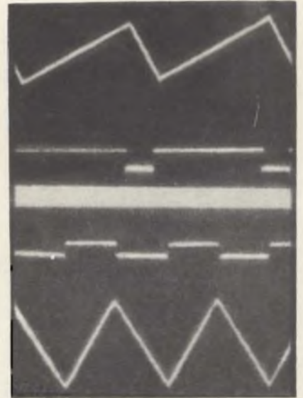
Fig. 10 - Oscillogrammi relativi al generatore di figura 9. In alto segnali a dente di sega, in basso segnali triangolari.
