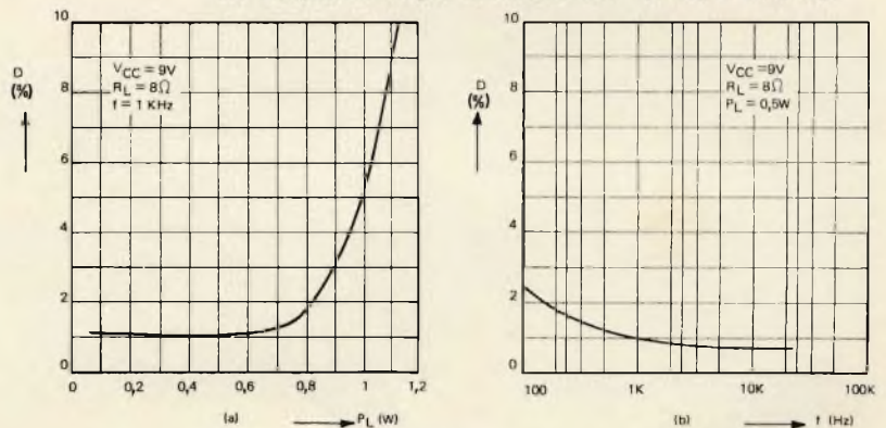
Fig. 26 - Distorsione tipica del circuito di fig. 25.
