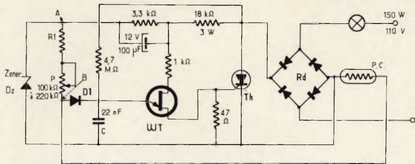
Fig. 14 - Circuito per il controllo della tensione di una lampada survoltata, impiegante un rettificatore controllato al silicio pilotato da un transistor a giunzione singola.
