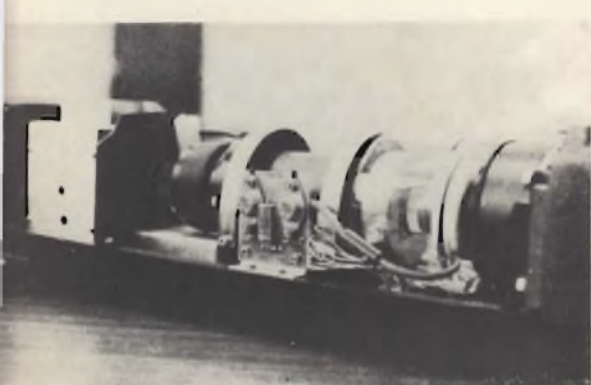
Fig. 3 - Fotografia illustrante il sistema ottico del laser impiegato nello interferometro.
