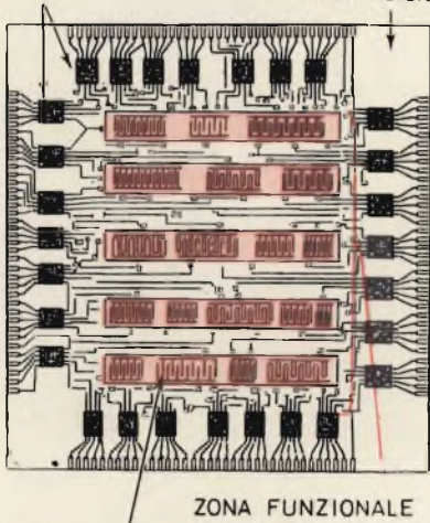
DISP. ELETTROACUSTICI
