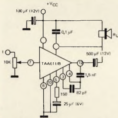
Fig. 29 - Impiego del TAA 611/B come amplificatore di B.F. ricevitori TV portatili. La potenza di uscita ottenibile è di 1,4 W con carico di 8 Ω di 0,8 W con carico di 16 Ω.
