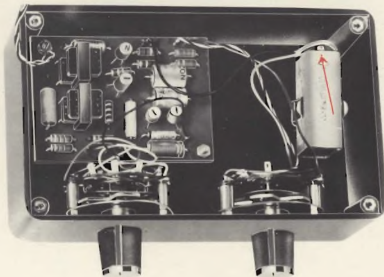
Fig. 4 - La freccia indica il punto dove si può verificare un processo di ossidazione (connettore per la pila).
