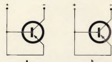
Fig. 13 - Misura della resistenza collettore-base a emittitore uniti.
