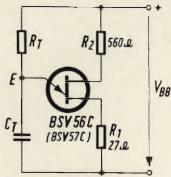
Fig. 7 - Schema elettrico di un semplice generatore di impulsi.
