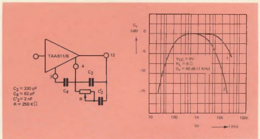
Fig. 23 - Controllo di tono per eliminazione delle alte frequenze. Circuito (23-a) e sua risposta in frequenza (23-b).
