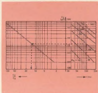
Fig. 22 - Grafico per la determinazione di C_2 e C_4 (fig. 21-c). Fissata la frequenza superiore della banda passante e la resistenza R_A , che determina il guadagno, si trova la capacità C_2 ed il rapporto C_2/C_4 .
