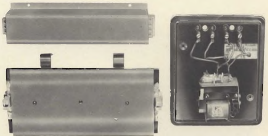
Fig. 3 - Ecco i componenti da impiegare per una illuminazione di emergenza (vedi schema di fig. 4).
