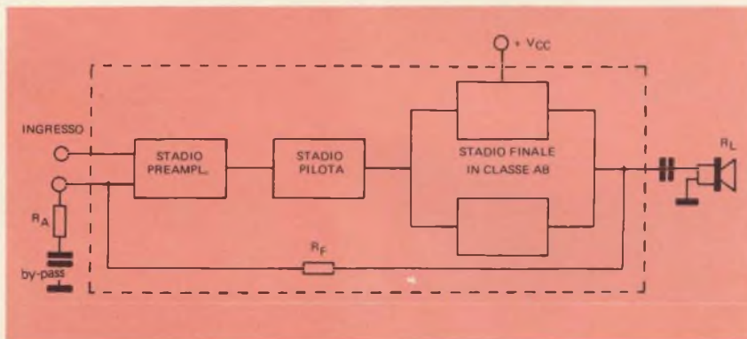
Fig. 1 - Schema a blocchi del TAA 611/B, amplificatore di bassa frequenza.
