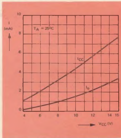
Fig. 13 - Corrente assorbita dal TAA 611/B in assenza di segnale ( I_{cc} ). Nel grafico è indicata anche la corrente assorbita dal solo stadio finale ( I_o ).
