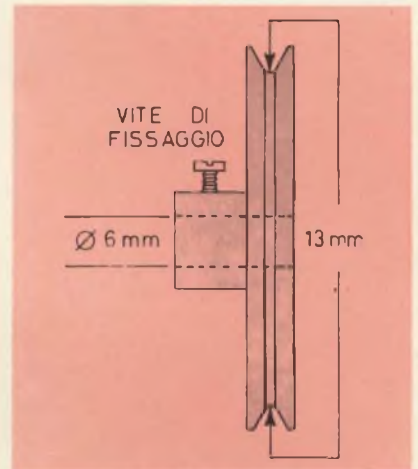
Fig. 10 - Aspetto della puleggia di trasmissione, vista di profilo, con un diametro riferito all'esempio fatto nel testo. Il diametro interno del foro passante deve essere adatto all'albero del potenziometro. Le pulegge di questo tipo sono reperibili presso la G.B.C. Italiana, tra i componenti meccanici per scale parlanti di ricevitori radio ecc.
