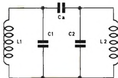
Fig. 11 - Circuiti accoppiati indirettamente per capacità.
