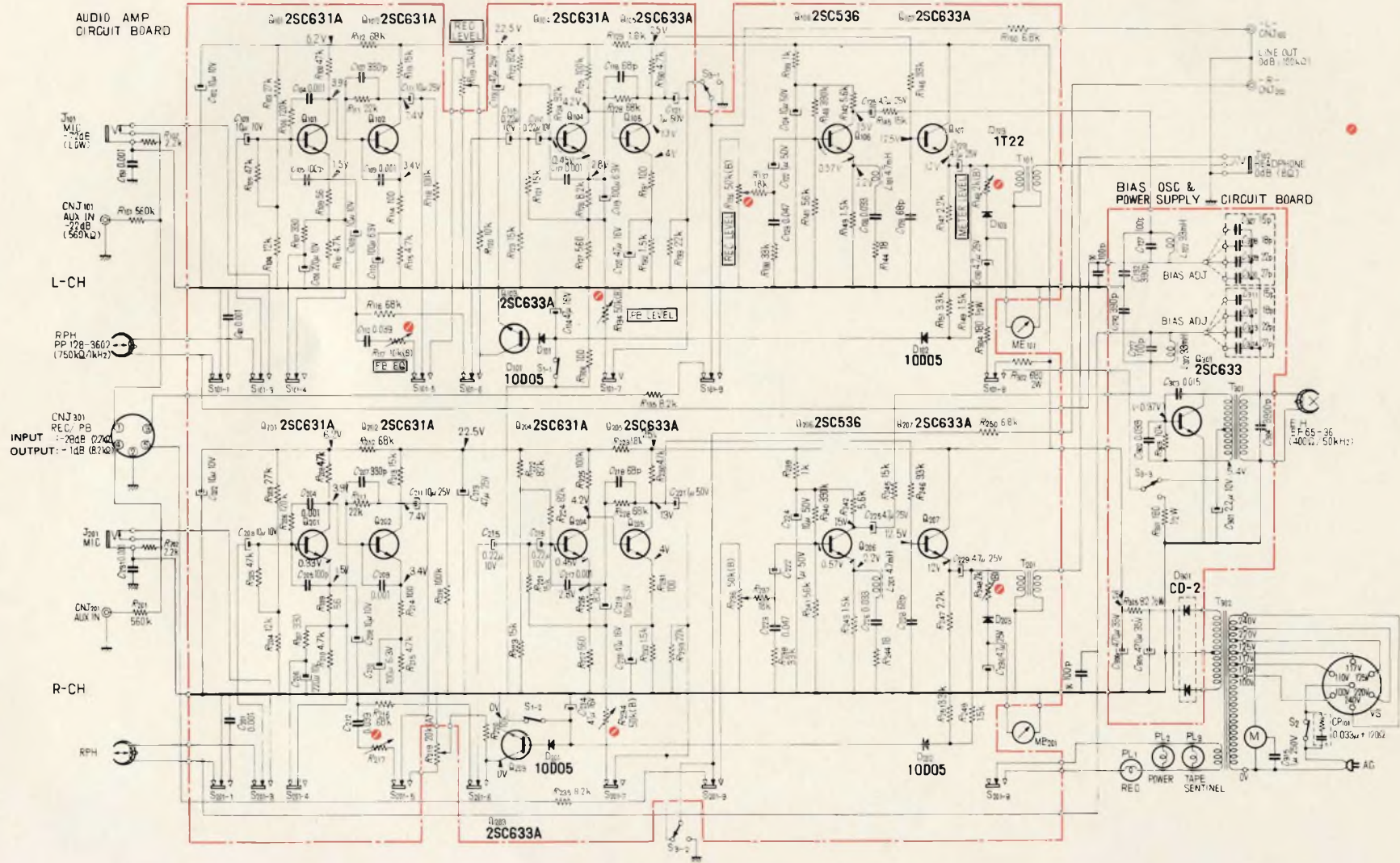
Fig. 2 - Schema elettrico del registratore Sony TC-127. I valori dei resistori e dei condensatori, salvo diversa precisione sono indicati rispettivamente in \Omega e in \mu F . I valori di tensione sono stati misurati con un voltmetro c.c. da 20 k \Omega/V in riproduzione senza segnale in ingresso. I valori di tensione in registrazione sono indicati fra parentesi ( ).
