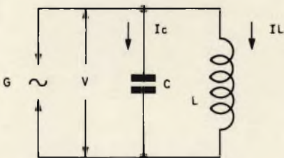
Fig. 13 - Esempio semplificato di un circuito oscillante.
