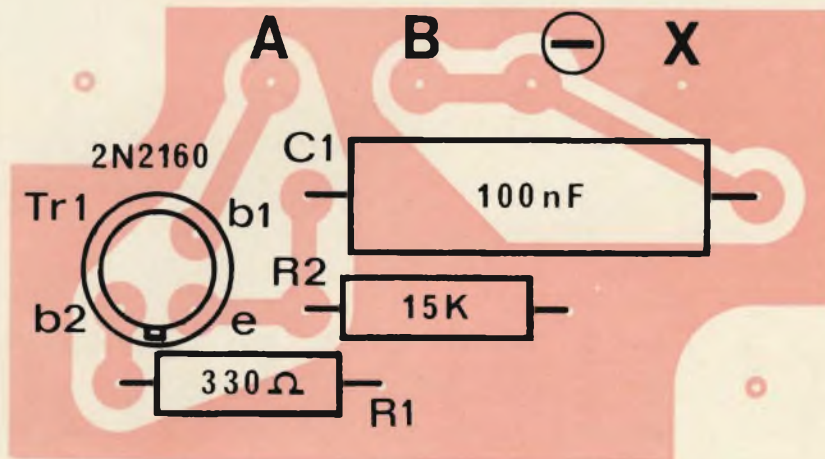
Fig. 2 - Disposizione dei componenti sulla basetta a circuito stampato del cercasfilì elettronico.
