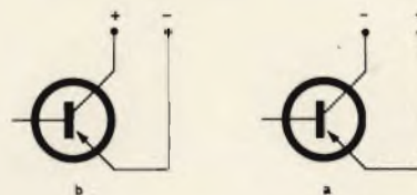
Fig. 12 - Misura della resistenza emettitore-collettore.
