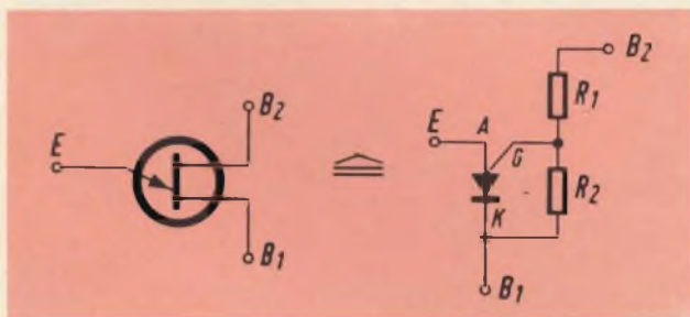
Fig. 5 - Circuito del transistor unigiunzione a programma con due resistenze, esso ha proprietà simili a quelle di un normale transistor unigiunzione.
