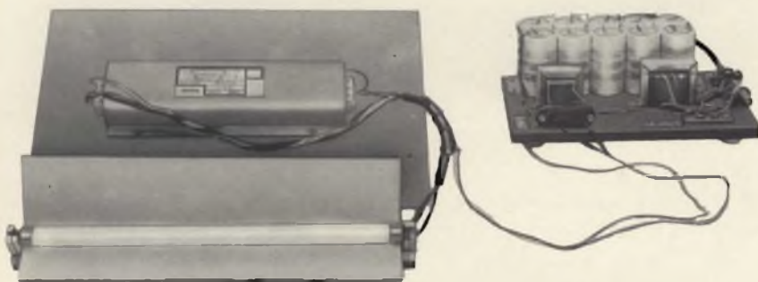
Fig. 5 - Ecco in funzione un dispositivo survoltore per l'alimentazione da batteria di una lampada fluorescente da 8 W. Si noti la piastra di alluminio di dissipazione su cui è montato il survoltore a transistori (8.000 Hz di funzionamento). Se si dispone di un qualsiasi elemento metallico di sufficiente superficie sull'impianto, questo potrà venire utilizzato con vantaggio al posto della piastra di dissipazione.
