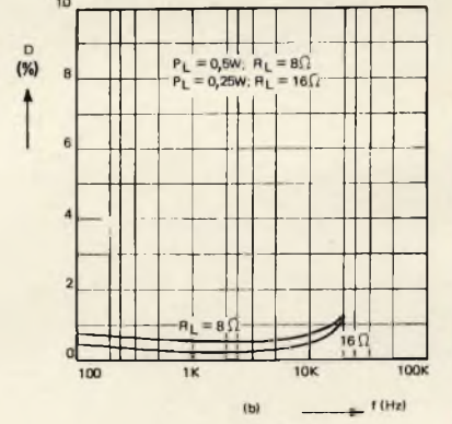
Fig. 30 - Distorsione tipica del circuito di fig. 29.
