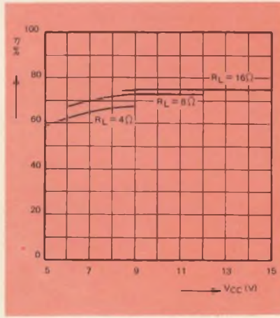
Fig. 12 - Rendimento del TAA 611/B nelle condizioni di massima potenza di uscita (distorsione 10%).
