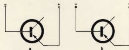
Fig. 11 - Misura della resistenza diretta e inversa base-emettitore.
