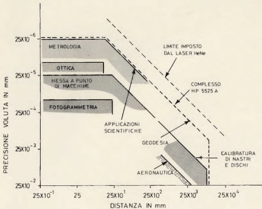
Fig. 6 - Grafico illustrante i diversi campi di applicazione dell'interferometro descritto.
