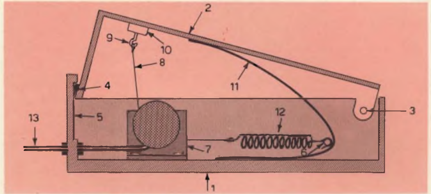
Fig. 9 - Disegno illustrante in sezione la struttura del pedale con trasmissione a puleggia, onde mettere in evidenza la posizione dei diversi componenti.
