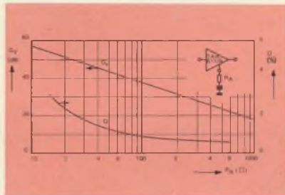
Fig. 16 - Variazione del guadagno di tensione G_V e della distorsione armonica totale D in funzione della resistenza R_L nel ramo di reazione.
