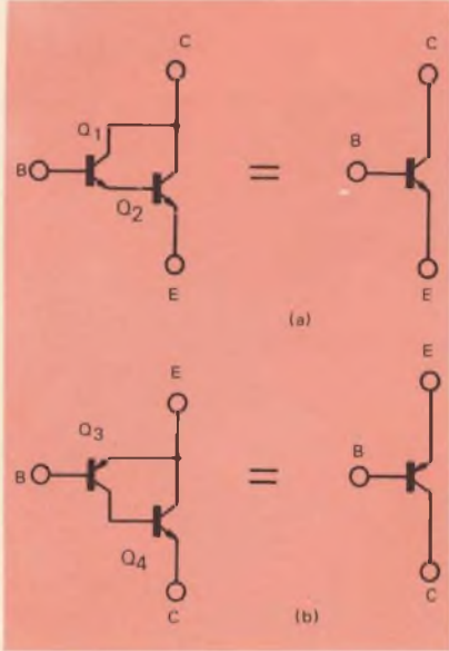
Fig. 5 - Transistori equivalenti dello stadio di uscita: NPN (3-a) e PNP (3-b).
