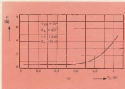
Fig. 17-a - Andamento tipico della distorsione armonica del TAA 611/B all'uscita.
