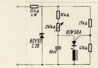
Fig. 11 - Circuito che può essere impiegato con notevoli vantaggi in sostituzione di quello racchiuso nel tratteggio in figura 10.
