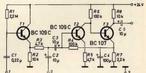
Fig. 1 - Schema elettrico di un preamplificatore per microfoni a bassa e ad alta impedenza. Grazie all'impiego dei transistori al silicio BC109C, il preamplificatore ha un valore di rumore estremamente basso. I resistori da R1 a R8 sono da 0,33 W, i condensatori elettrolitici da C2 a C5 hanno una tensione di lavoro di 15 V.
