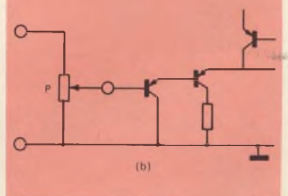
Fig. 18 - Polarizzazione in ingresso del TAA 611/B, utilizzando una resistenza R_G (18-a) e lo stesso potenziometro del volume (18-b).
