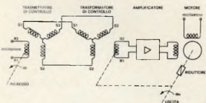
Fig. 8 - Schema elementare di applicazione del Synchro 18CT6a.
