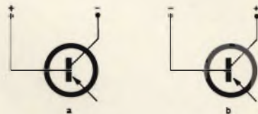
Fig. 10 - Misura della resistenza inversa e diretta collettore-base.
