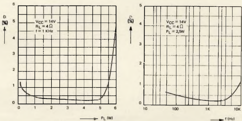
Fig. 32 - Caratteristiche del circuito di fig. 31.
