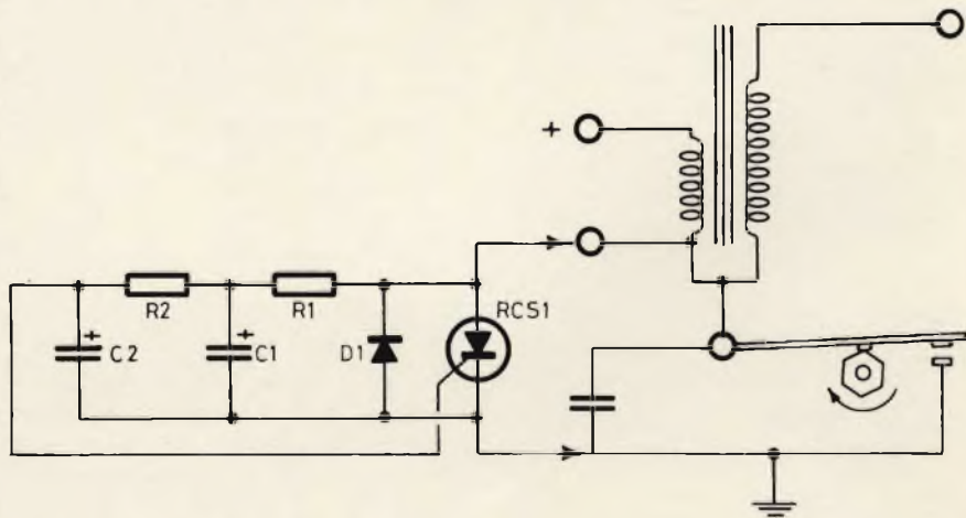
Fig. 4 - Circuito elettrico del dispositivo di accensione, costituito dalla bobina e dalle puntine, con l'aggiunta del sistema di prolungamento della durata del punto morto.
