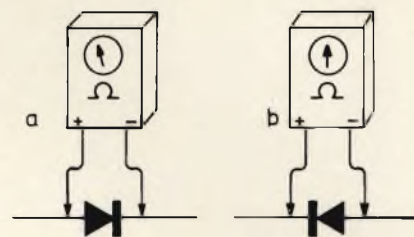
Fig. 9 - Misura della resistenza diretta (a), e della resistenza inversa (b) di un diodo.
