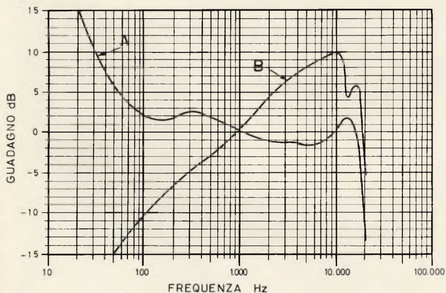
Fig. 2 - Curve di responso ottenibili con l'intervento delle cellule correttive: A per testina piezoelettrica con carico di 1\text{ M}\Omega , e B per testina magnetica.
