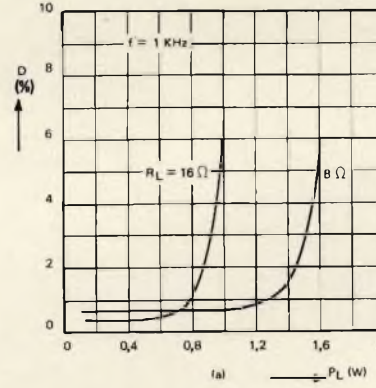
Fig. 30 - Distorsione tipica del circuito di fig. 29.
