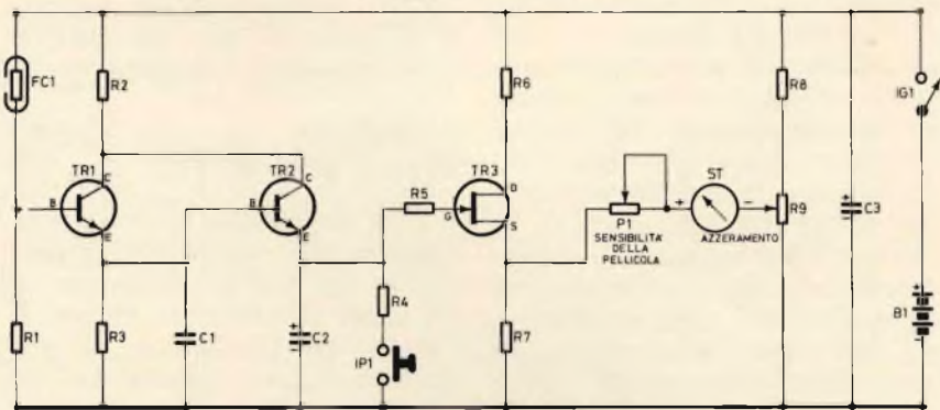
Fig. 2 - Circuito elettrico completo del fotometro: TR1 e TR2 costituiscono un amplificatore ad accoppiamento diretto, mentre TR3 ed ST costituiscono un voltmetro elettronico ad altissima resistenza interna. In pratica, il circuito permette di misurare la carica che si accumula in C2, ogni qualvolta la fotocellula FC1 viene eccitata da un lampo di luce.
