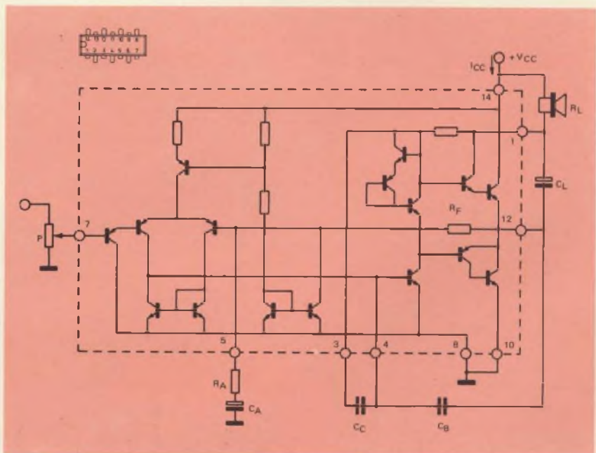
Fig. 8 - Schema elettrico completo del TAA 611/B e dei relativi componenti esterni.
