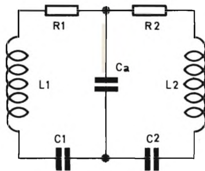
Fig. 10 - Circuiti accoppiati direttamente tramite capacità.
