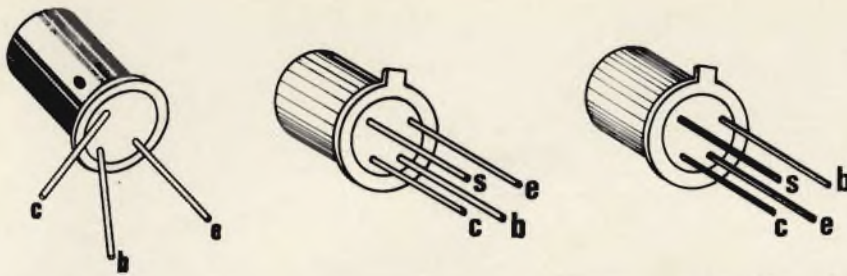
Fig. 14 - Frequentemente un punto colorato sta ad indicare la posizione del terminale di collettore, ma in certi transistori una piccola sporgenza è posta in corrispondenza del terminale di base o di emettitore. Talvolta esiste un quarto terminale (s): è collegato allo schermo.
