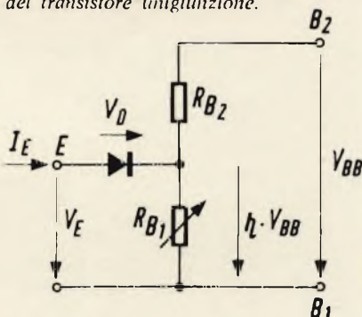
Fig. 1b - Circuito equivalente semplificato del transistor unigiunzione.
