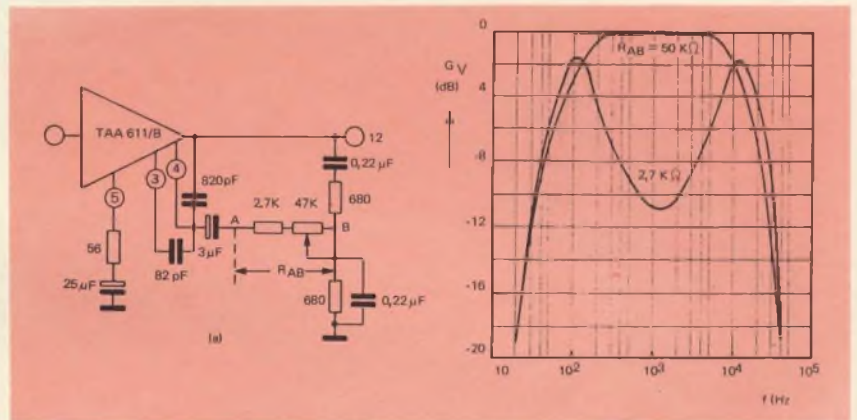
Fig. 23 - Controllo di tono per eliminazione delle alte frequenze. Circuito (23-a) e sua risposta in frequenza (23-b).
