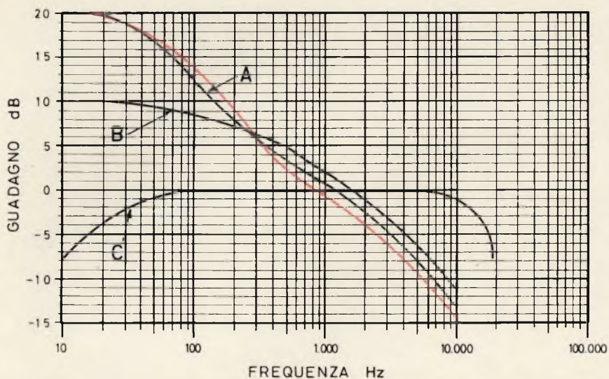
Fig. 7 - Grafico illustrante le curve globali di responso del preamplificatore, sia per testine magnetiche (curve A e B, differenziate a seconda del valore di R5), sia per testine piezoelettriche (curva C), rispetto alla curva teorica RIAA, riprodotta in colore.
