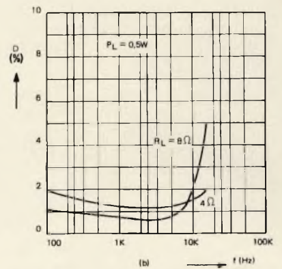
Fig. 28 - Distorsione tipica del circuito di fig. 27.
