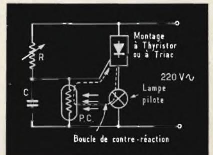
Fig. 15 - Esempio di metodo di regolazione dell'intensità luminosa di una lampada survoltata, mediante un circuito di controreazione eccitato della stessa luce prodotta.
