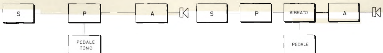
Fig. 2 - Lo stesso principio di cui alla figura 1 può essere sfruttato per controllare il tono, attenuando le alte o le basse mediante un potenziometro azionato a pedale, facente capo al preamplificatore.
