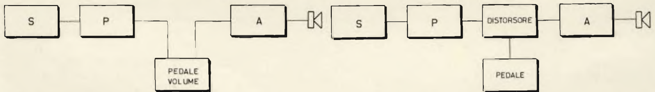
Fig. 1 - Schema a blocchi illustrante l'applicazione di un comando a pedale tra il preamplificatore (P) e l'amplificatore (A), per controllare il volume dei suoni prodotti dall'altoparlante e provenienti dallo strumento S.
