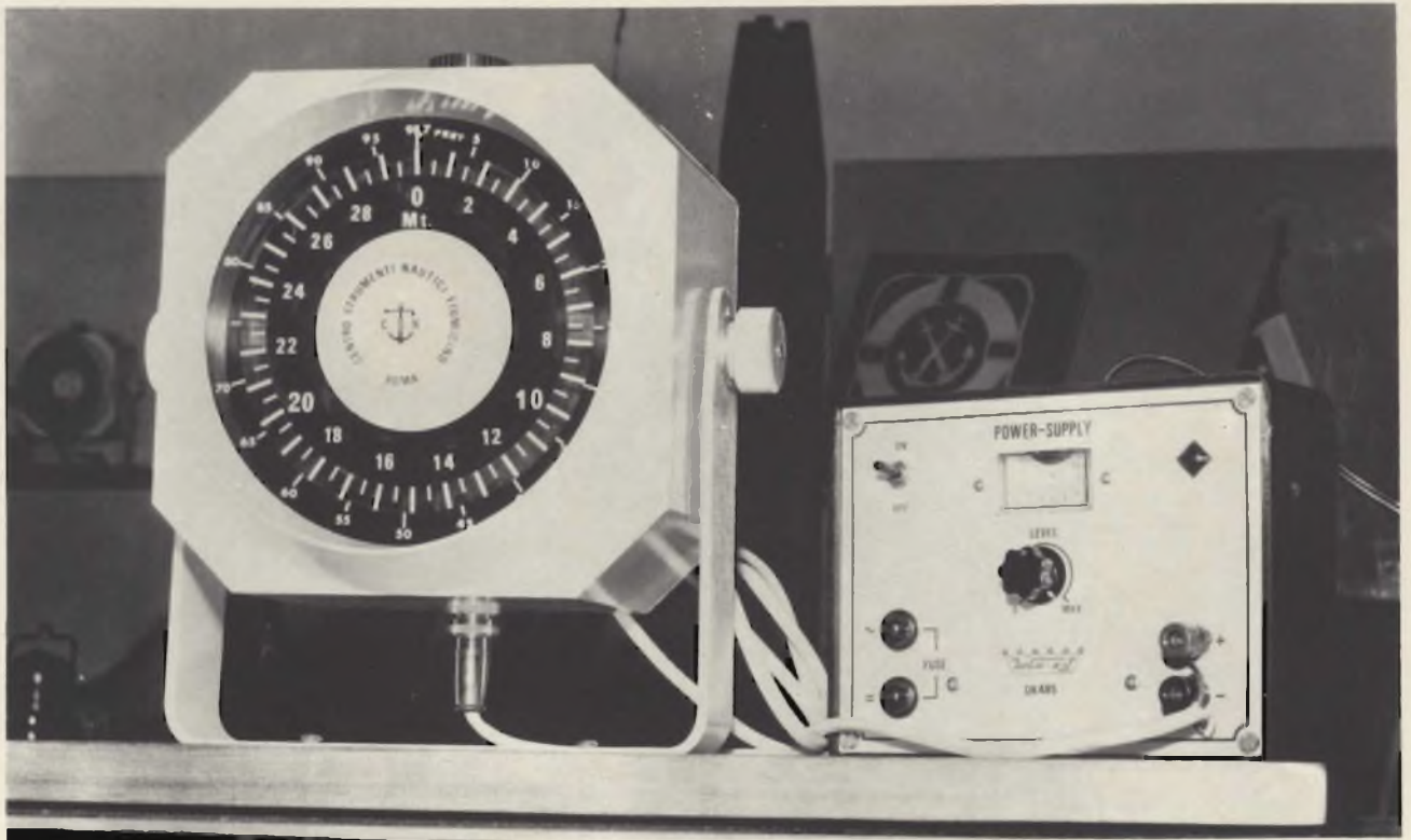
Fig. 5 - Ecoscandaglio ultrasonoro ECS-5069-1 del centro strumenti Nautici-Fiumicino, alimentato a 12 V.c.c. mediante l'alimentatore HIGH-KIT UK 485.
