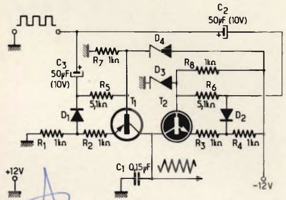
Fig. 9 - Schema di un generatore di segnali a transistori lineari.
