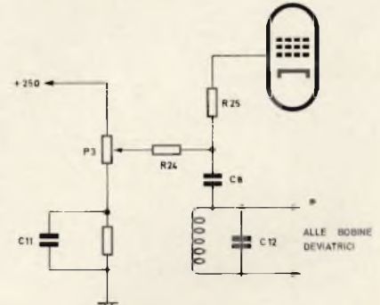
Fig. 11 - Sezione relativa al controllo di luminosità di un televisore.
