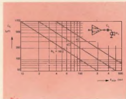
Fig. 20 - Grafico per la determinazione della capacità di accoppiamento dell'altoparlante C_1 .
