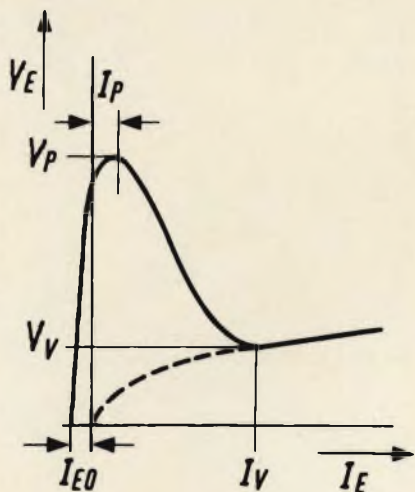
Fig. 3 - Curva caratteristica illustrante il valore di cresta I_p , V_p e il valore minimo I_v , V_v .
