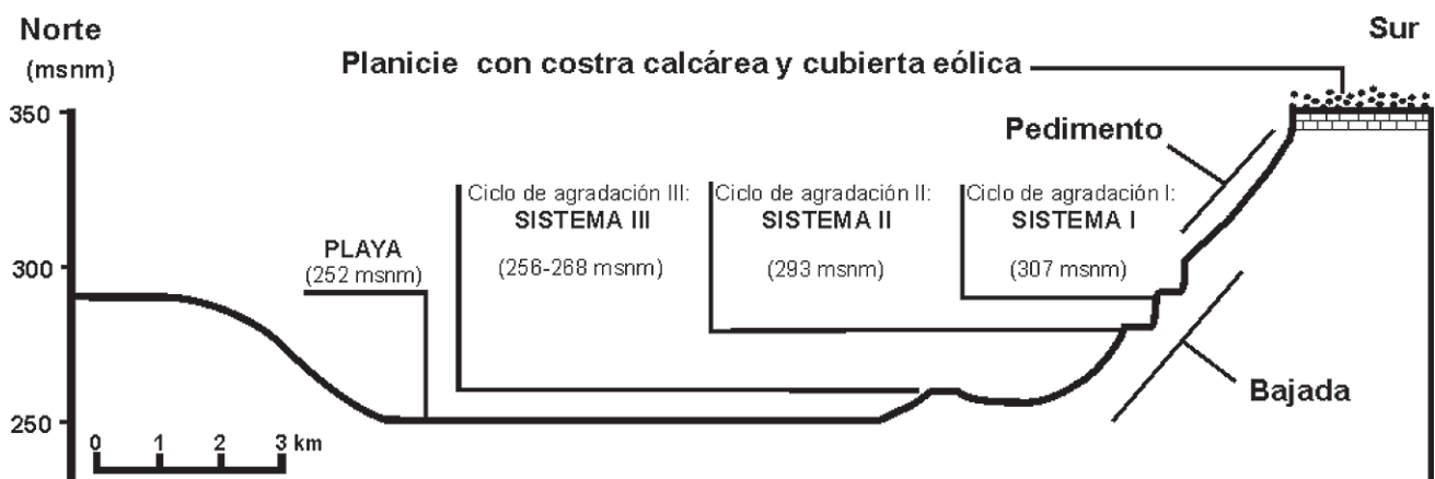
Figura 11. Esquema longitudinal N-S del Bajo del Durazno. Se ilustra la posición de los tres sistemas de elevaciones (escala vertical exagerada) interpretados como sendos niveles de piedemonte.
