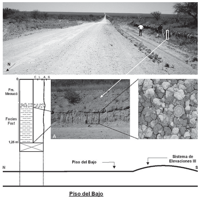
Figura 10. Piso del Bajo: esquema transversal de la sección y fotos de las litofacies. Relaciones estratigráficas.
