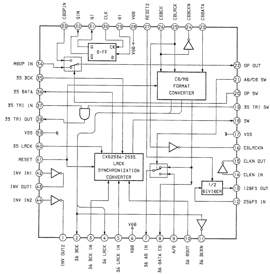
IC251 CXD8640Q
