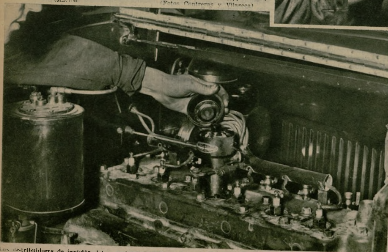
Los distribuidores de ignición deben revisarse con frecuencia, así como las bujías, cuyo aparente buen estado determina averías y "pannes" frecuentes
