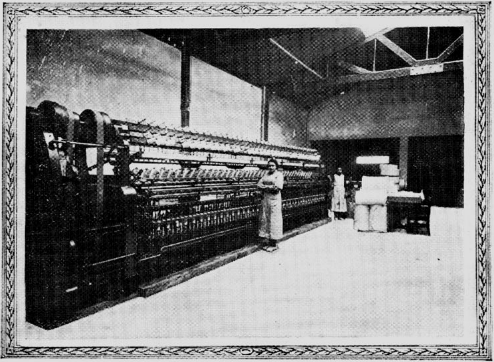
Sección torcedura de hilados de fantasía.
