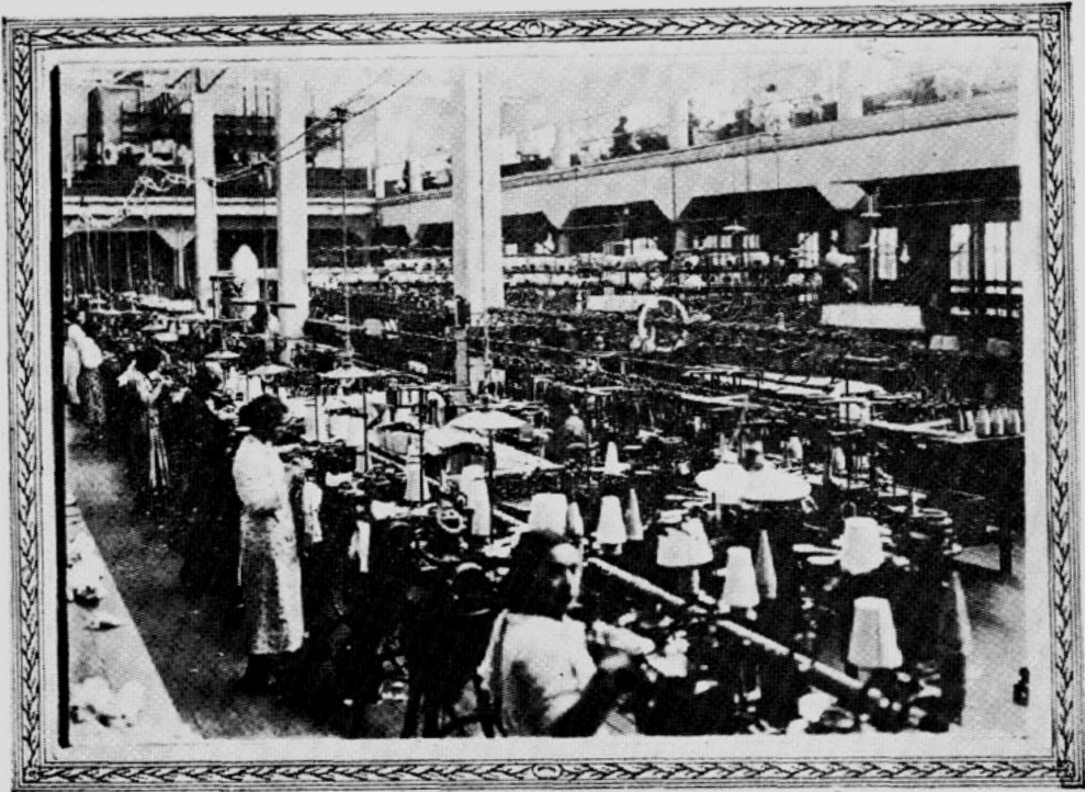
Sección Calcetería.
