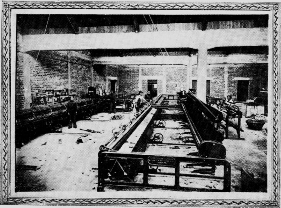
Sección Selfactine.
