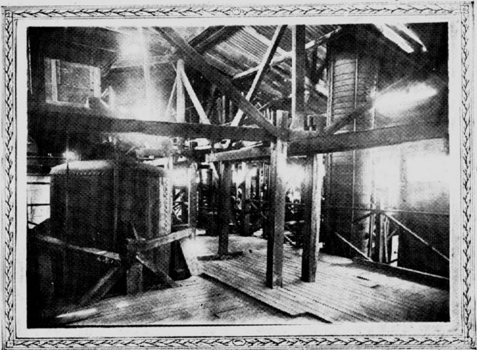
Sección Cocimiento
