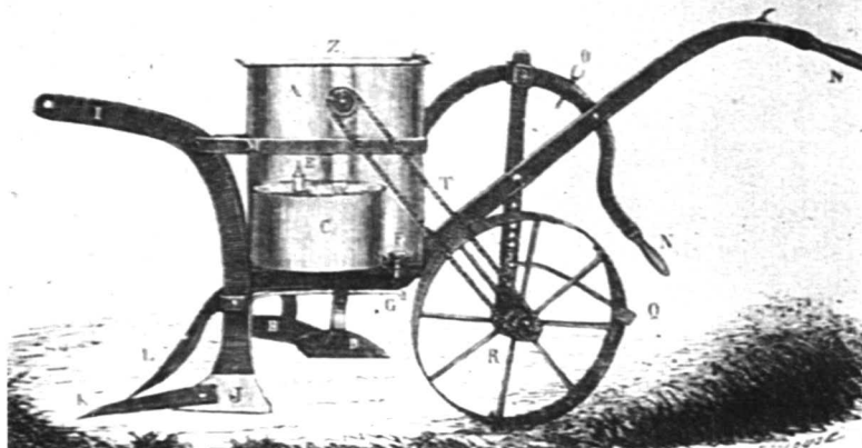
Fig. 49: Arado sulfurador.
