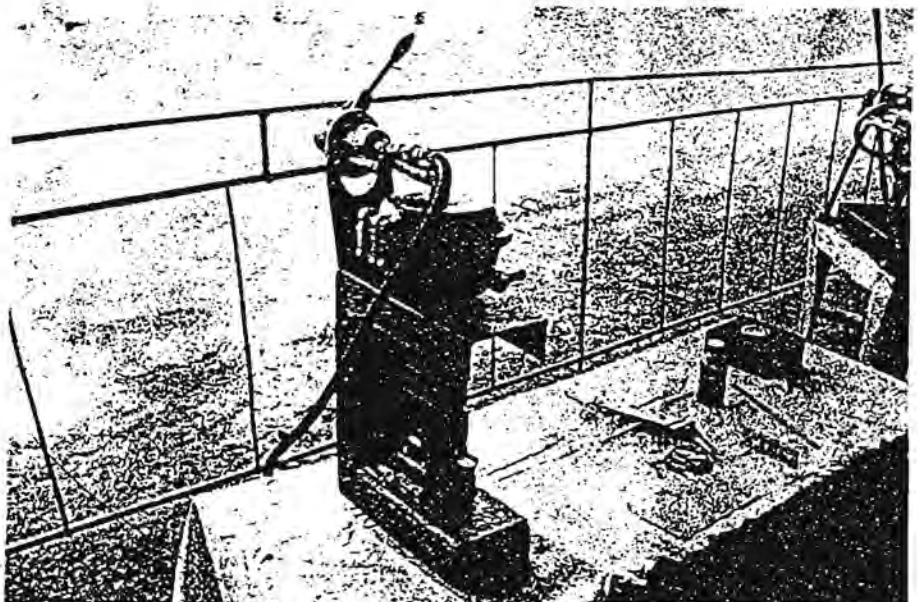
Máquina para fabricar remaches utilizados en los taxis y ómnibus. Cienfuegos, Cienfuegos.
