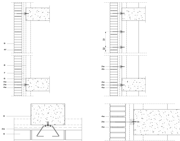
Figura 5.4: Sección vertical. Detalle de fijación de anclaje GEOANC® a forjado o pilar.
