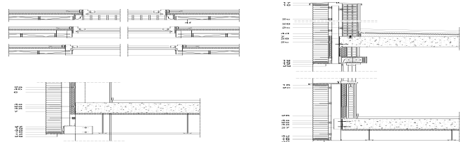
Figura 5.21c: Sección horizontal por hueco. Jamba mediante pieza especial.
