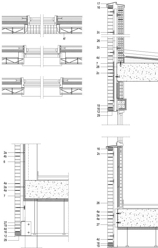
Figura 5.19: Dintel de hueco y coronación. Hoja exterior e interior ancladas a perfil metálico tubular resistente.
