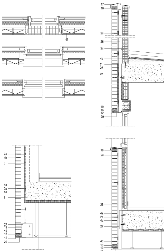
Figura 5.20: Arranque sobre cargadero fijado a perfil metálico resistente.
