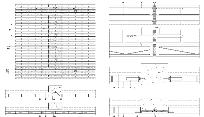
Figura 5.9: Sección horizontal. Fijación de anclaje GEOANC® 0 a pilar.
