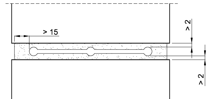
Figura 5.14: Recubrimiento mínimo de armaduras.
