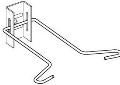
Figura 2.4: Anclaje GEOANC® 3.
