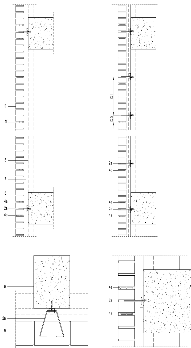
Figura 5.1: Sección vertical del sistema.
