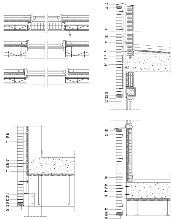
Figura 5.22: Arranque sobre cargadero fijado a pilar mediante ángulos.
