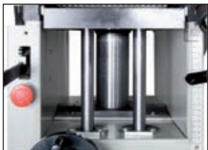
Το τραπέζι για το ξεχόνδρισμα στηρίζεται σε 3 στιβαρούς οδηγούς για μέγιστη σταθερότητα
