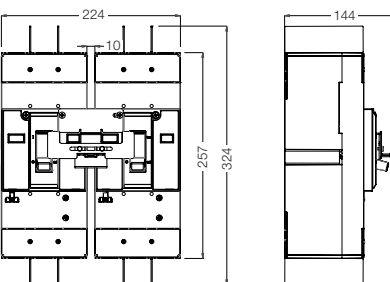
Tamaño 400 3P + BLIM DWB400 3P
