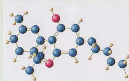
Representación de una molécula de THC.
