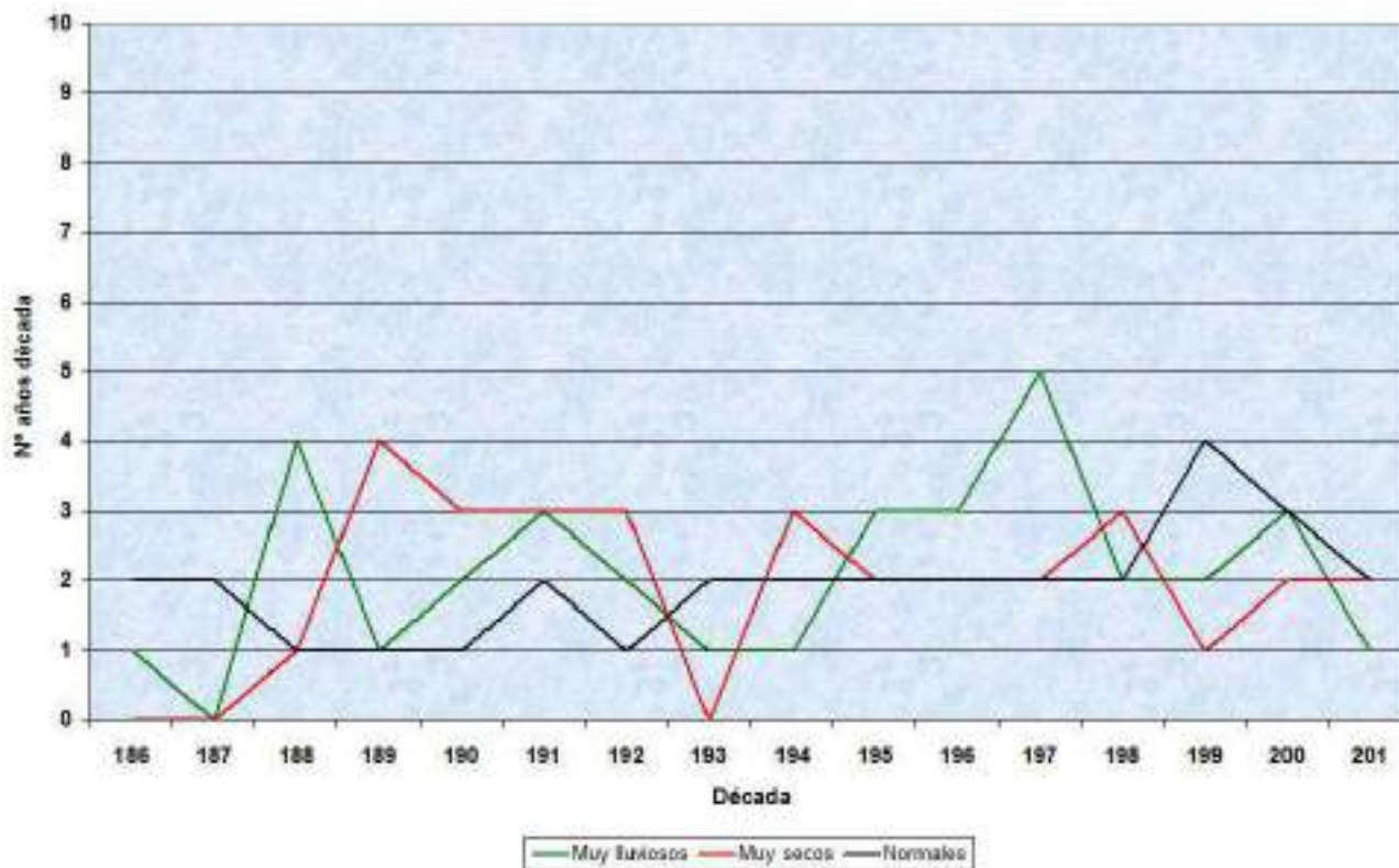
Gráfica 35: Evolución temporal de los años decenales de precipitación anual muy lluviosos, muy secos y normales:
