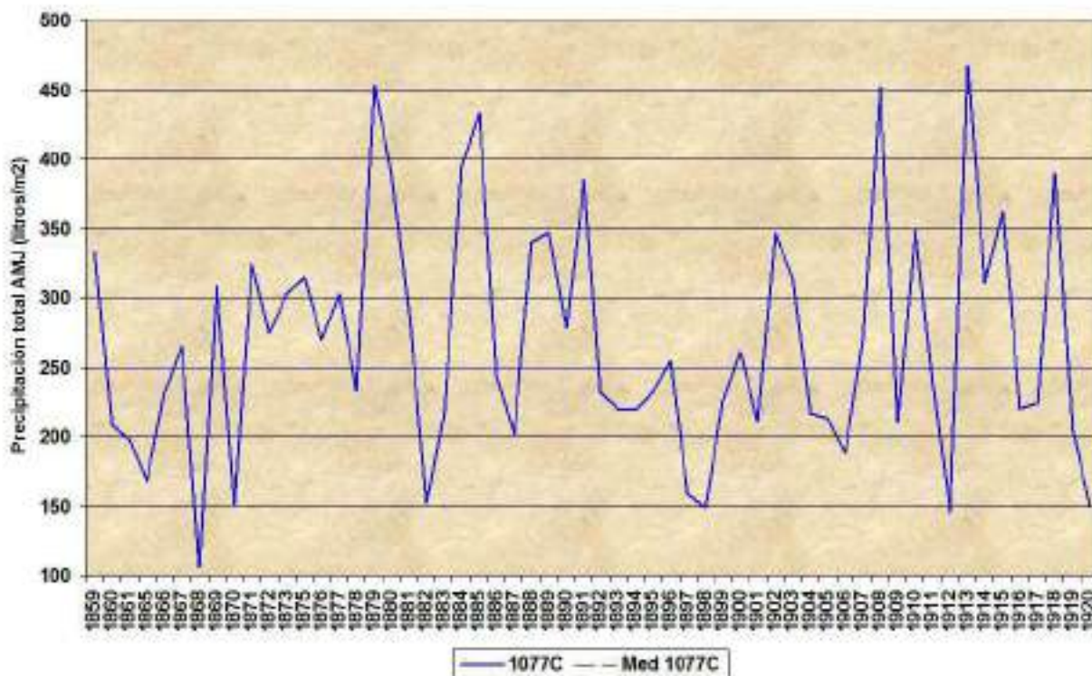
Gráfica 103: Precipitación total AMJ creciente de 1077C 📍:
