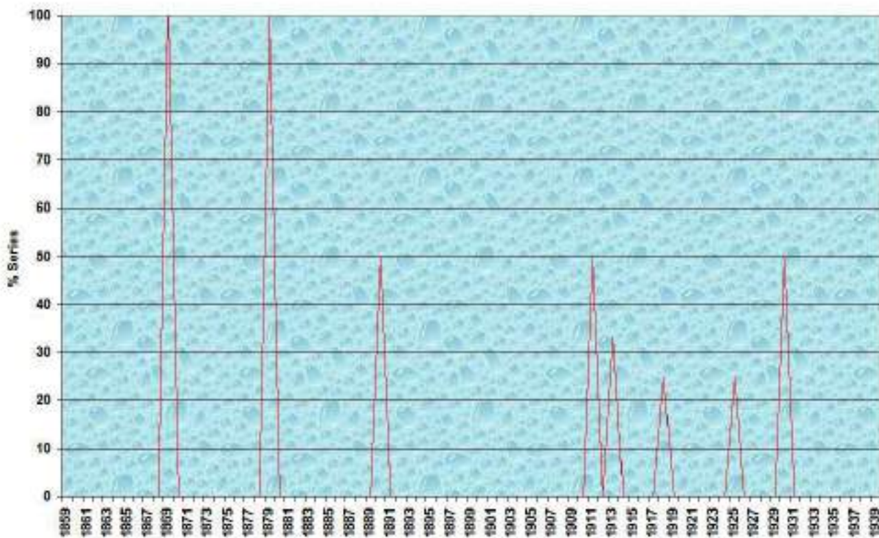
Gráfica 50: Evolución temporal del % de MAM muy lluviosos (150 % mediana) de 1859 a 1939:
