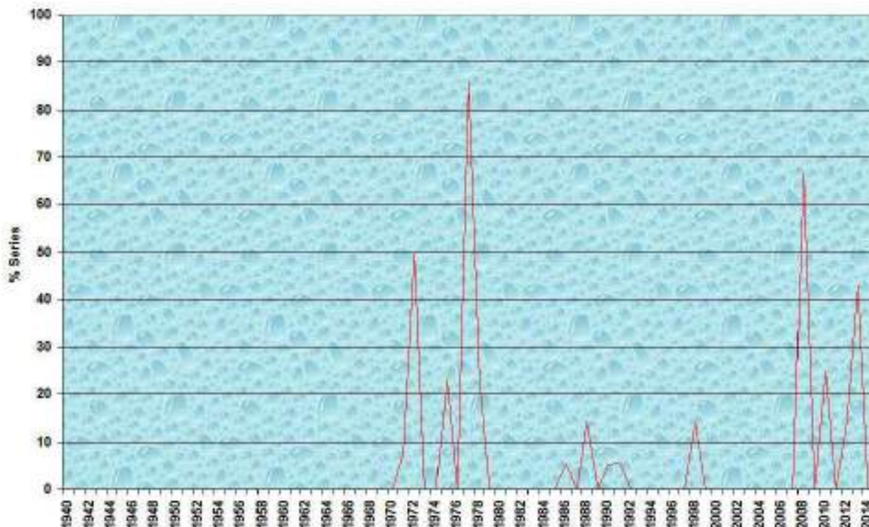
Gráfica 68: Evolución temporal del % de AMJ muy lluviosos (150 % mediana) de 1940 a 2014:
