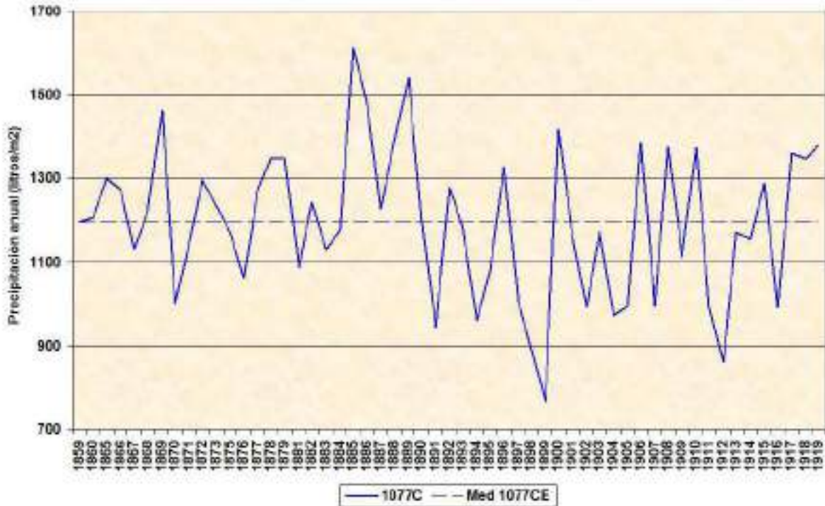
Gráfica 87: Precipitación total anual creciente de 1077C ♡:
