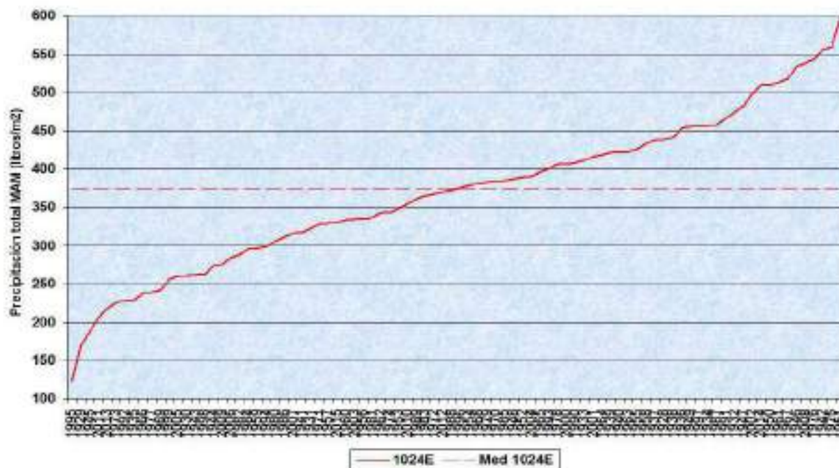
Gráfica 91: Precipitación total MAM creciente de 1024E 📍:
