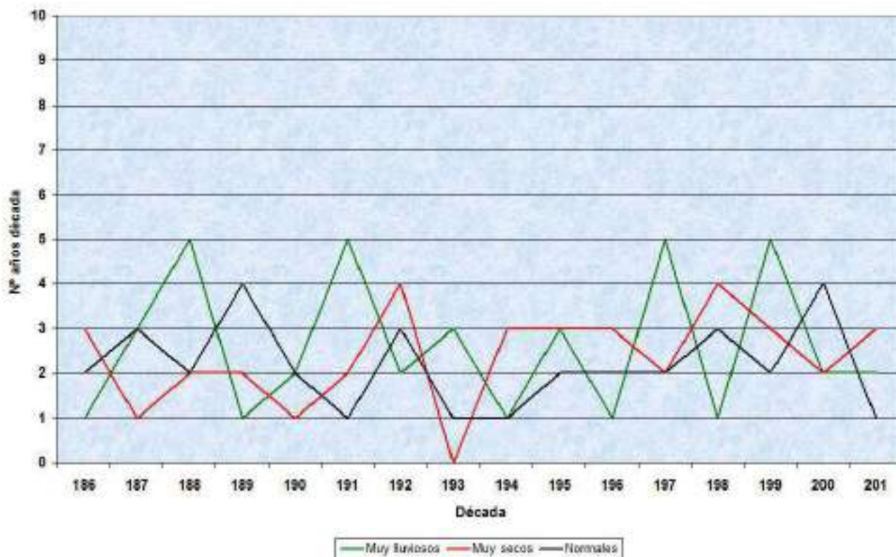
Gráfica 75: Evolución temporal de los años decenales de precipitación AMJ muy lluviosos, muy secos y normales:
