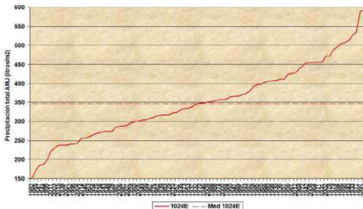
Gráfica 99: Precipitación total AMJ creciente de 1024E 🇨🇷:
