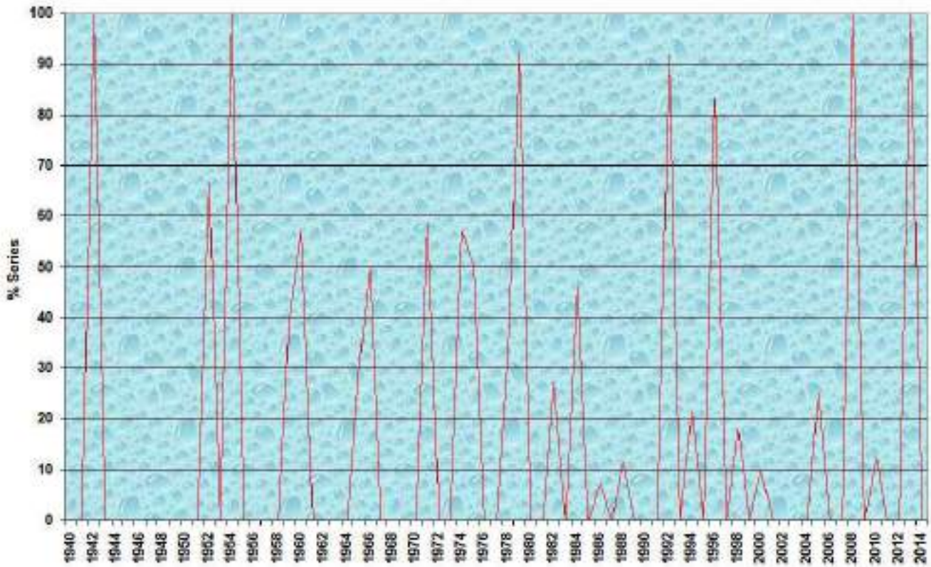
Gráfica 24: Evolución temporal del % de años lluviosos (quintil superior) de 1940 a 2014:
