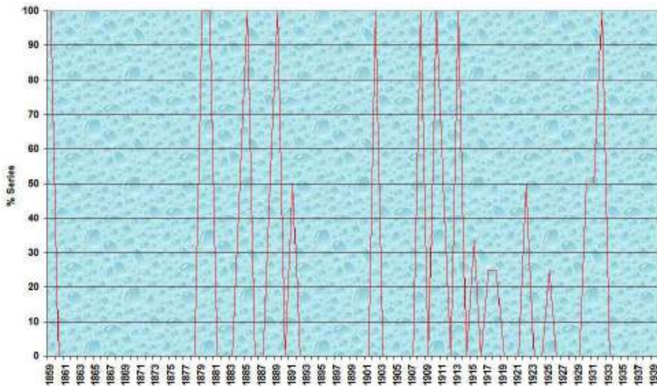
Gráfica 67: Evolución temporal del % de AMJ muy secos (67 % mediana) de 1859 a 1939:
