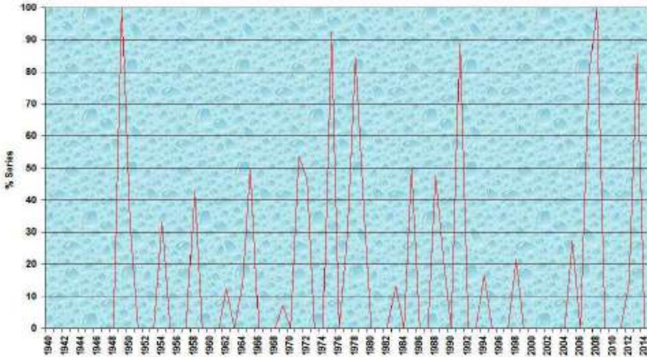
Gráfica 37: Evolución temporal del % de MAM secos (quintil inferior) de 1940 a 2014:
