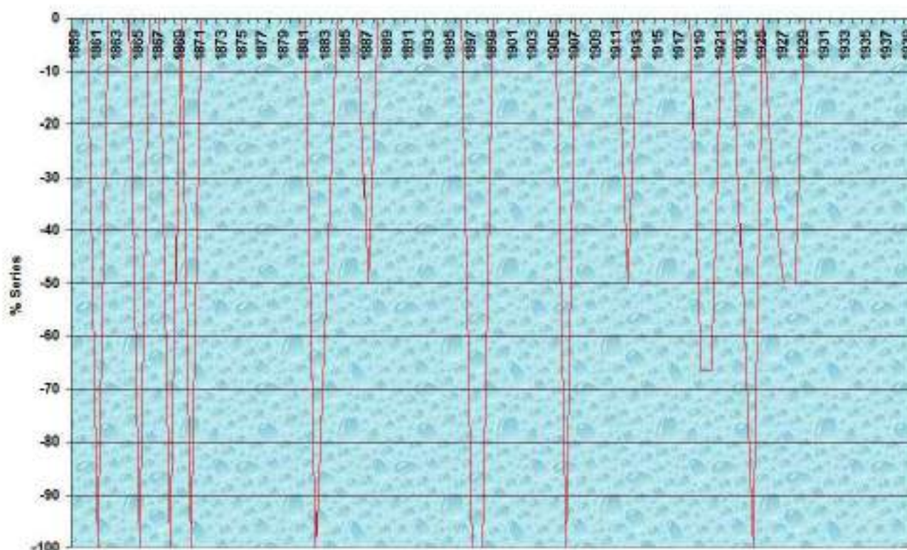
Gráfica 63: Evolución temporal del % de AMJ secos (80 % mediana) de 1859 a 1939:
