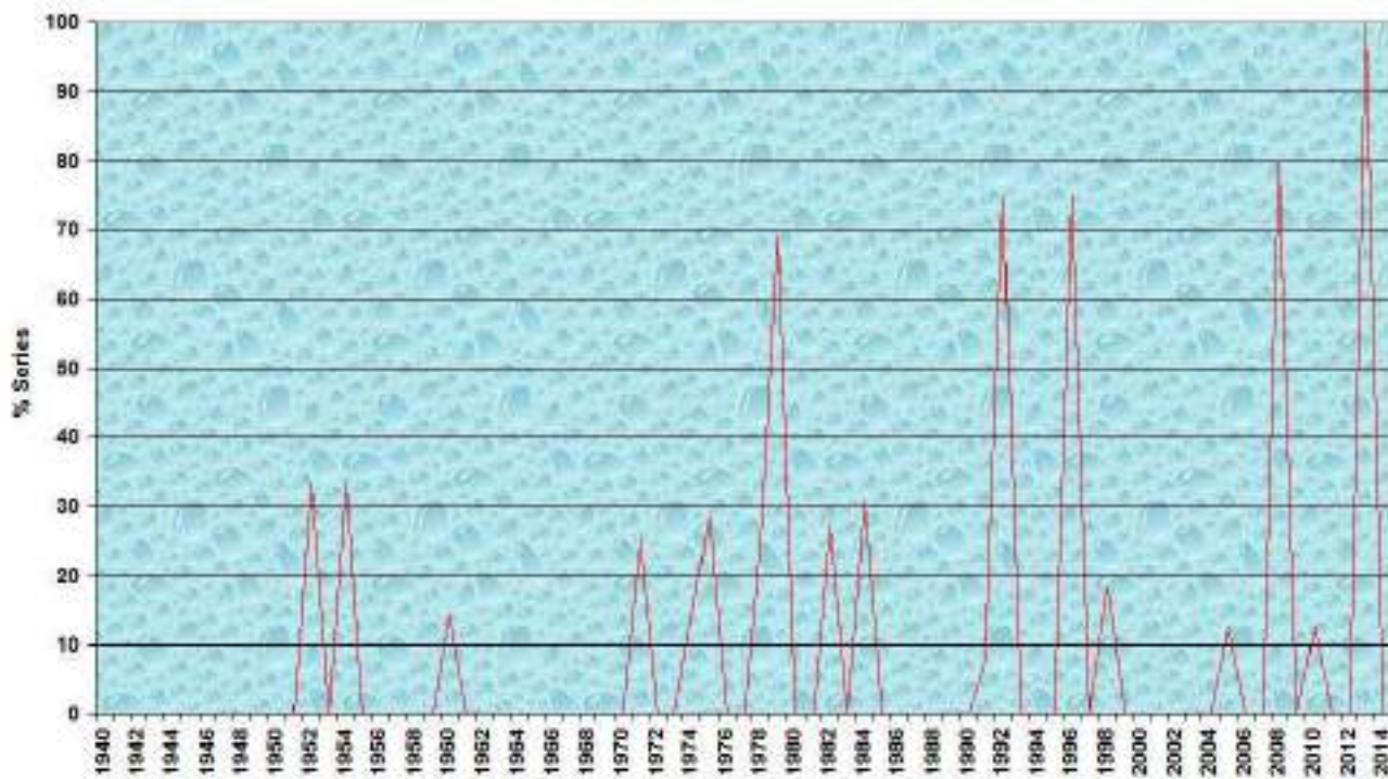
Gráfica 28: Evolución temporal del % de años muy lluviosos (120 % mediana) de 1940 a 2014:
