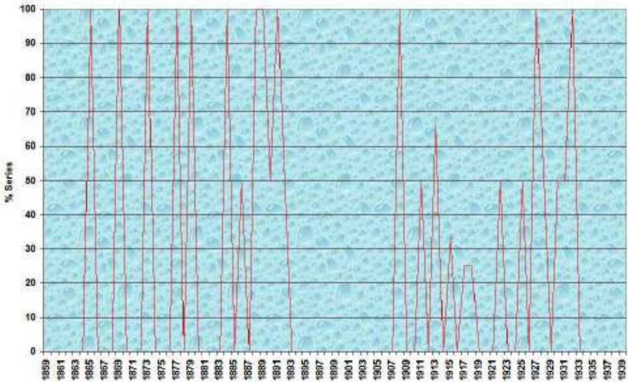
Gráfica 42: Evolución temporal del % de MAM lluviosos (120 % mediana) de 1859 a 1939:
