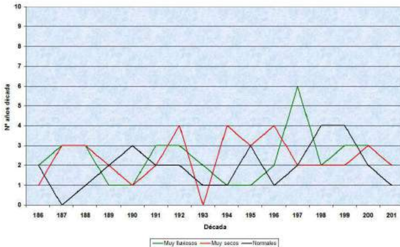
Gráfica 55: Evolución temporal de los años decenales de precipitación MAM muy lluviosos, muy secos y normales:
