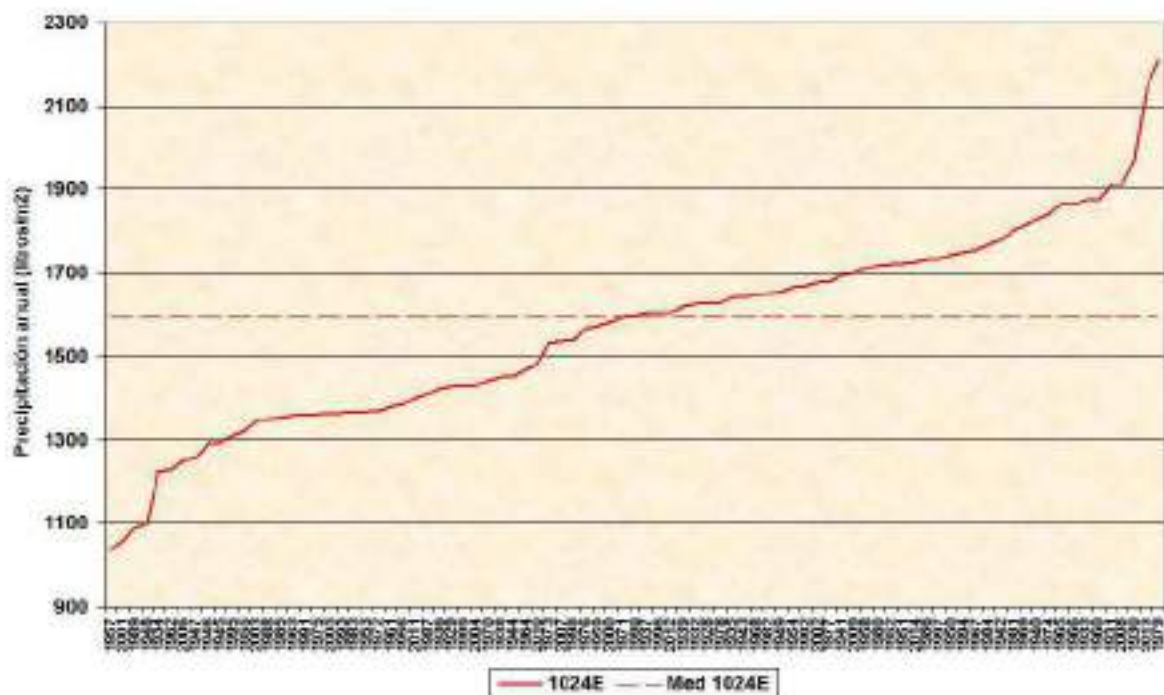
Gráfica 83: Precipitación total anual creciente de 1024E 🇪🇸:
