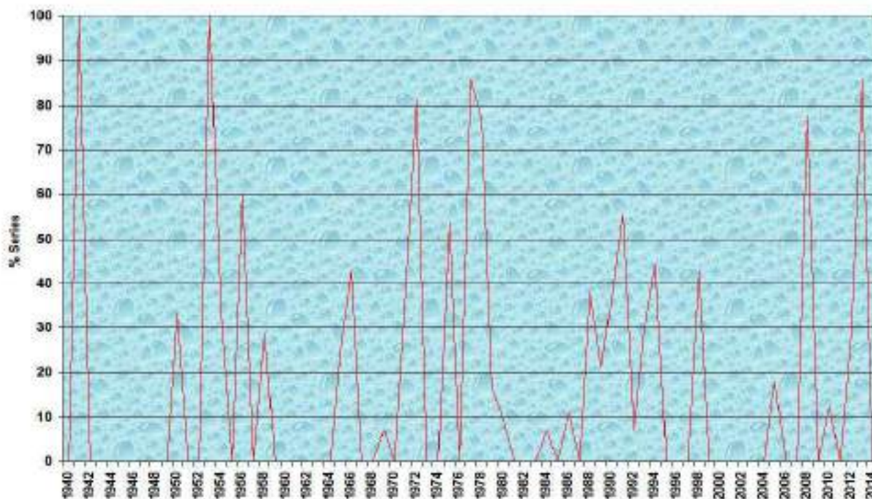
Gráfica 57: Evolución temporal del % de AMJ secos (quintil inferior) de 1940 a 2014:
