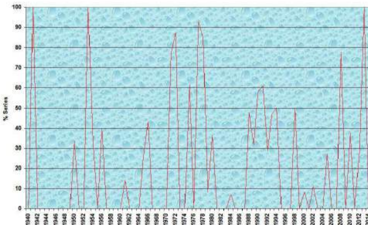
Gráfica 60: Evolución temporal del % de AMJ lluviosos (120 % mediana) de 1940 a 2014:
