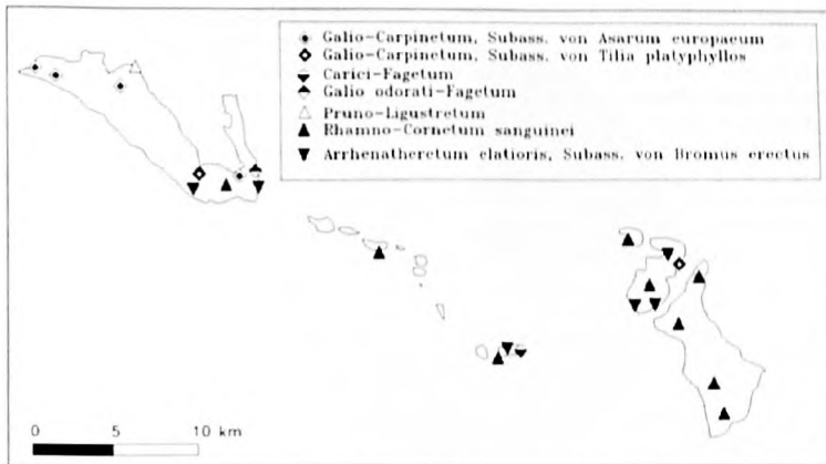
Abb. 2. Verbreitungskarte ausgewählter Pflanzengesellschaften im USG (1. Teil)
