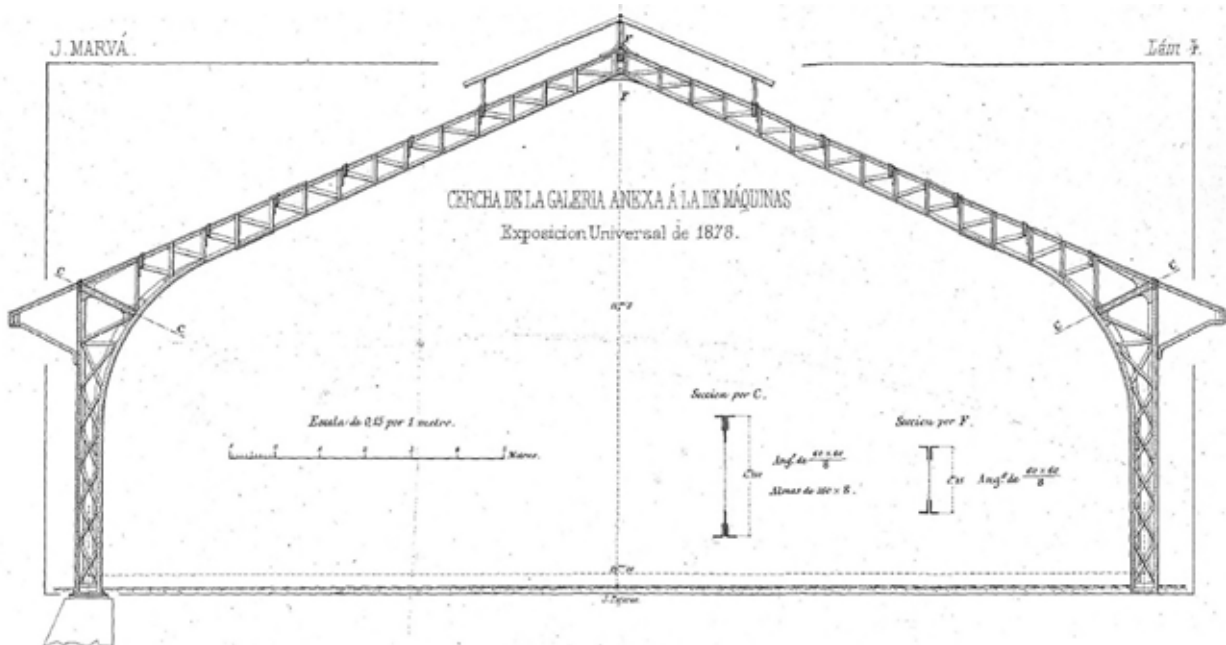
Cercha
