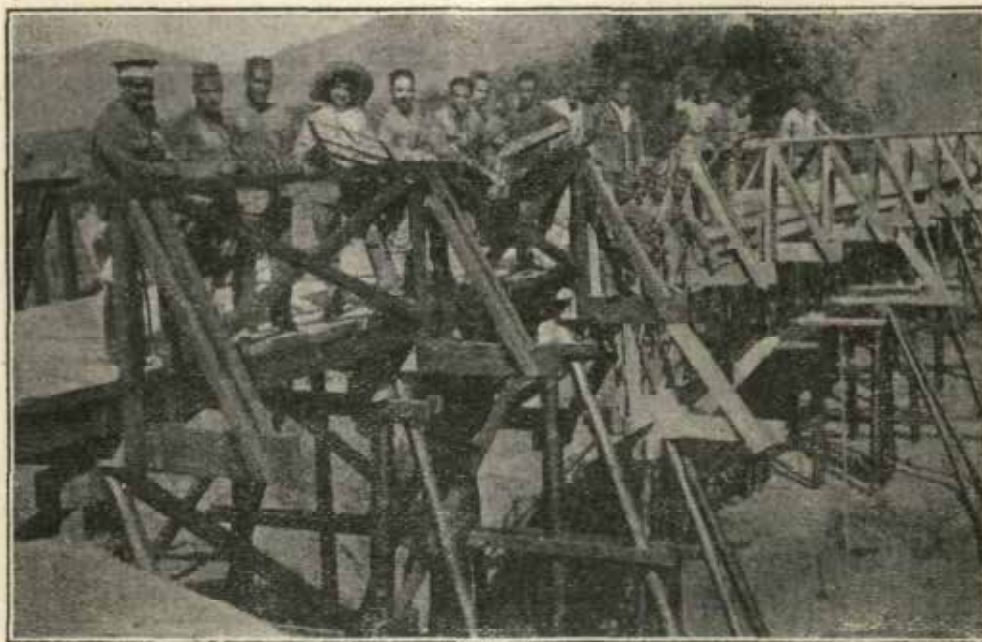
Puente viaducto en el camino de Anual. Terminación de los trabajos.
