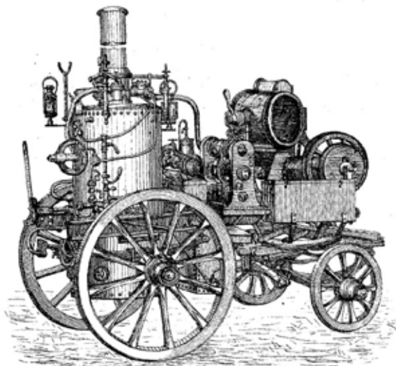
Proyector de luz de campaña
