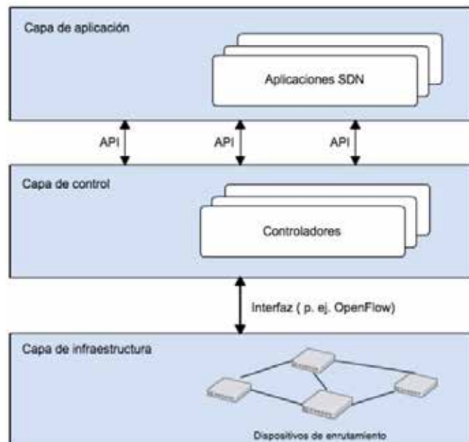
Arquitectura general de las SDN
