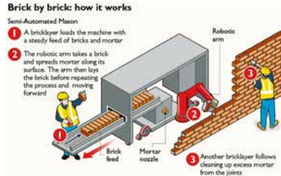
Robot de construcción de tabiquería de ladrillo "Semi-Automated Mason" (SAM100)
