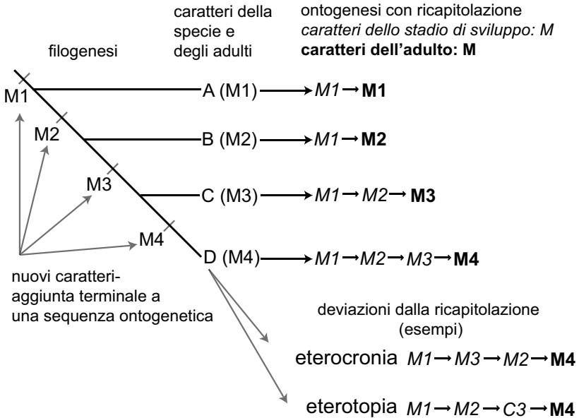
Figura 1.7. Aggiunte terminali nell'evoluzione delle sequenze ontogenetiche conducono alla ricapitolazione ontogenetica. Tuttavia ci sono delle deviazioni da questo modello. Modificato da Wägele (2005).
