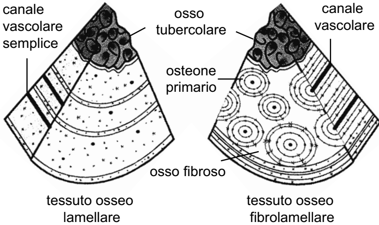
Figura 4.2. Rappresentazione schematica di due tipi fondamentali dell'istologia delle ossa. Questi sono generalmente presenti nei «rettili» ectotermi (a sinistra) e negli uccelli e mammiferi endotermi (a destra). Modificato da Chiappe (2007).
