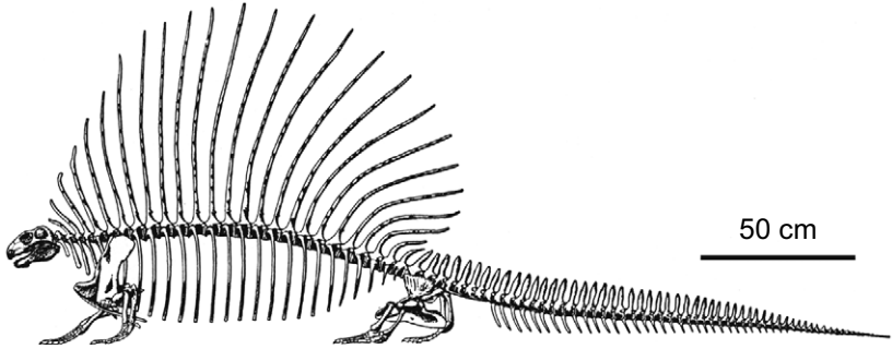
Figura 5.4. Il «pelicosaurio» Edaphosaurus boanerges . Modificato da Romer e Price (1940) e Sander (1994).
