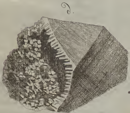
c. d. Chrystaller.
