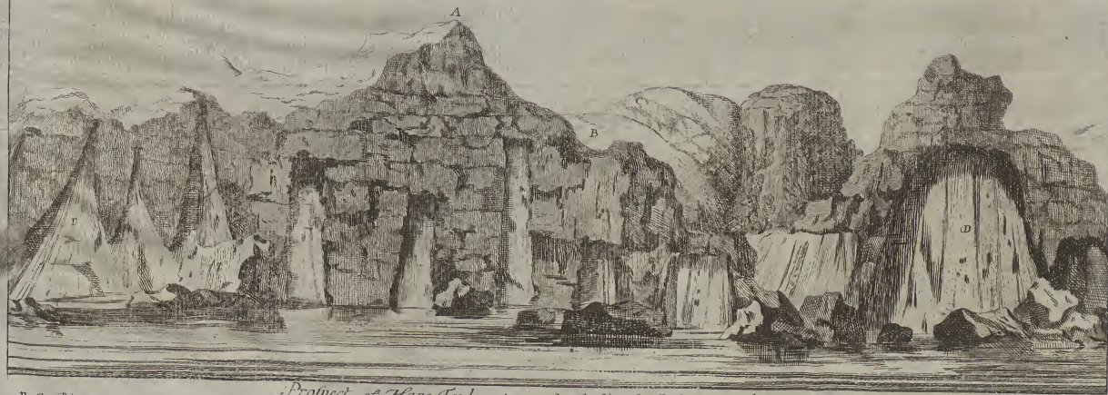
Prospect of Hage-Lavlen, A. og andre høvliggende Bardestrands Fjælde. B. C. Bierg; Iage. kaldede Toor og Høllur, fordi de seer ud som Høller eller Skæbe med Afdelinger. D. Fjeld-Skræde E. Rød hardet jord, som gierne findes mellem Lagene.
