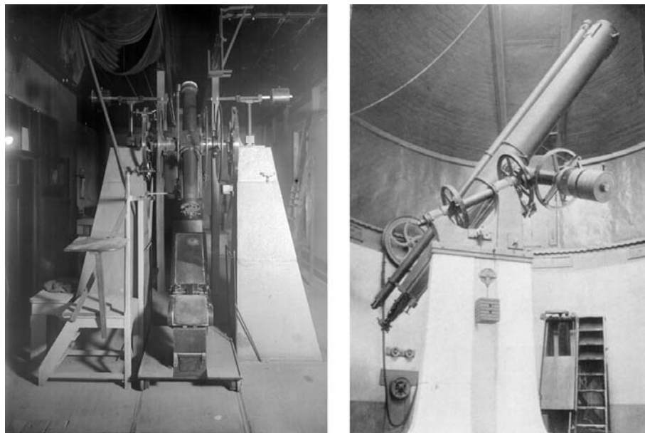
Figura 8. Izquierda: Círculo Meridiano Repsold Derecha: El “Gran Ecuatorial” con la montura Warner & Swasey, montado en la vieja cúpula. (Archivo OAC. Digitalizadas por los autores)
