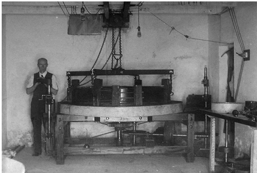
Figura 24. James Oliver Mulvey junto al espejo de 1,5 metros en el banco de trabajo, en el taller de óptica recién inaugurado (marzo 1914). (Archivo OAC, digitalizada por los autores)
