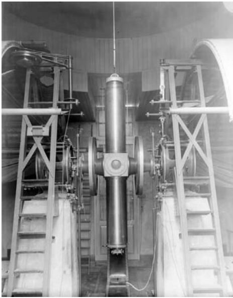
Figura 15. Nuevo Círculo Meridiano Repsold de 190 mm de diámetro. (Archivo OAC)
