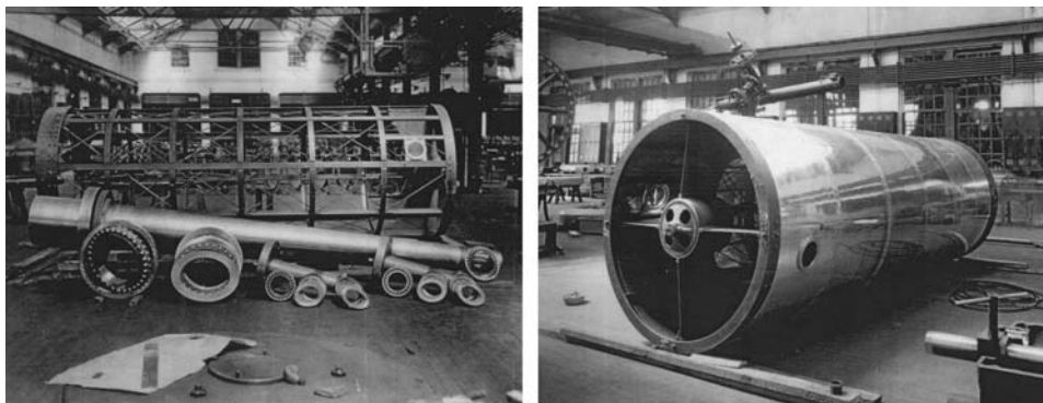
Figura 30. Izquierda: El telescopio en la fábrica Warner and Swasey de Cleveland, EE.UU.. Se aprecia el eje polar y los rodamientos. Derecha: El tubo del telescopio armado, cerrado con chapas de aluminio. (The Warner and Swasey Collection, Kelvin Smith Library, Case Western Reserve University)
