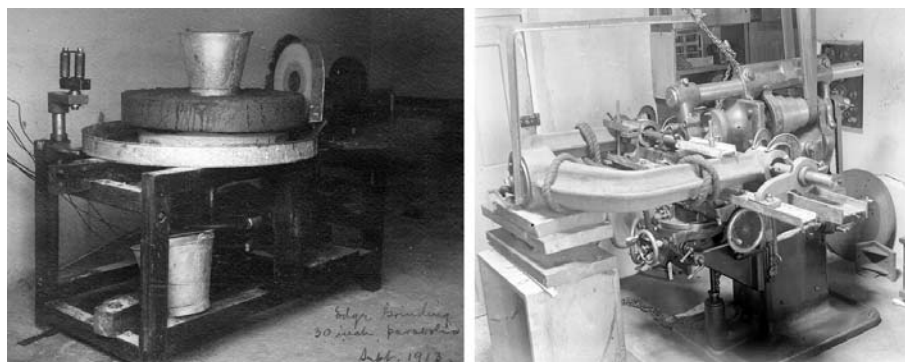
Figura 25. Izquierda: El espejo de 75 cm en el banco de trabajo, 1913. Derecha: La horquilla del telescopio en el taller mecánico del Observatorio, 1917. (Archivo OAC, digitalizadas por los autores)
