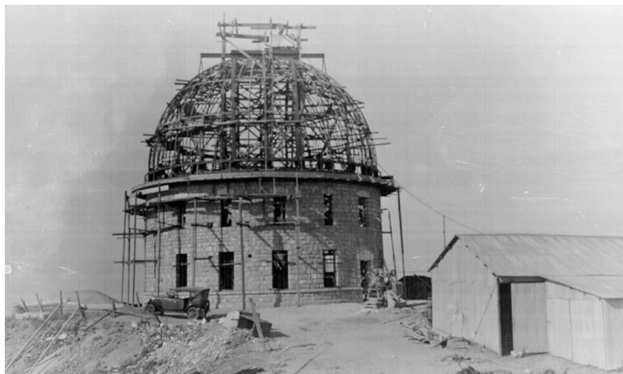
Figura 29. La cúpula de Bosque Alegre en pleno proceso de armado, 1930. (Archivo OAC)
