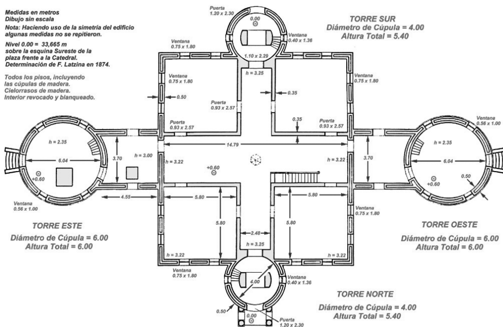
Figura 6. Plano de la primera sede del Observatorio Nacional Argentino, 1871. (Paolantonio y Minniti 2001)
