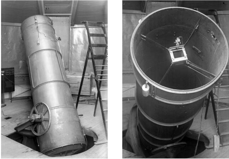
Figura 26. Izquierda: El reflector de 75 cm terminado, montado en la vieja cúpula, 1917. Derecha: Detalle del porta placa del telescopio. (Archivo OAC, digitalizadas por los autores)
