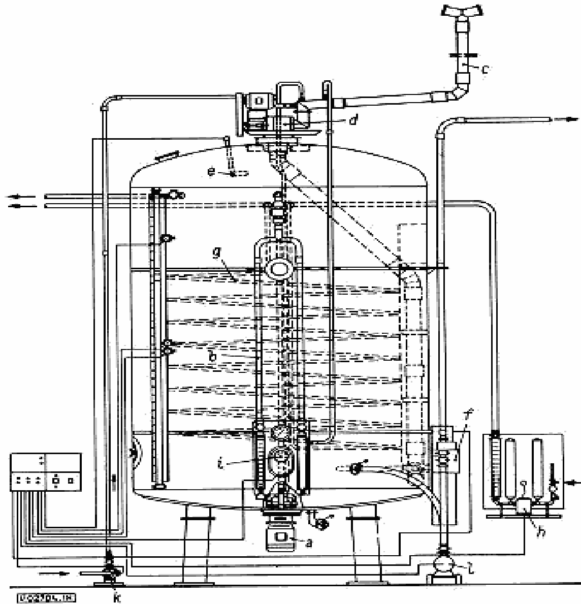
Figura 4. Corte transversal de um acetificador para elaboração de vinagre pelo método com fermentação acética submersa; a- turbina de ar; b- compensador de ar; c- dispositivo para coletar líquido de condensação; d-e- dispositivo para controlar a formação de espuma; f- dispositivo para medir o álcool; g- serpentina para refrigeração; h- dispositivo para refrigeração; i- termômetro; j- bomba para entrada do vinho; k- bomba para retirada do vinagre.
