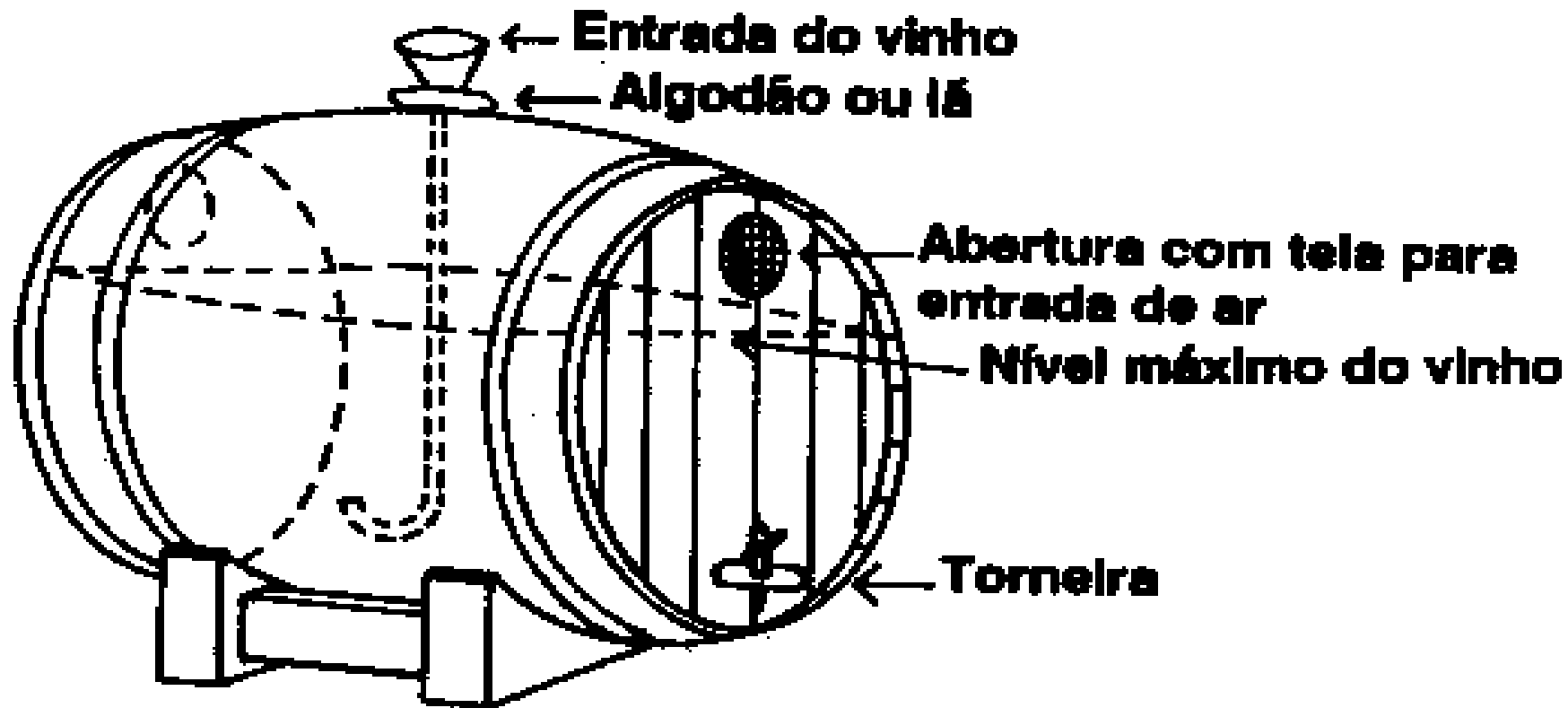
Figura 1. Recipiente utilizado para elaboração de vinagre pelo processo Orleans.
