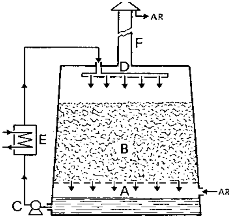
Figura 2. Corte transversal de um acetificador com suporte poroso; A) grade; B) maravalha de madeira; C) bomba para movimentação do vinho em processo de acetificação; D) dispersor do vinho; E) refrigerante de água; F) dispositivo de condensação de vapores.
