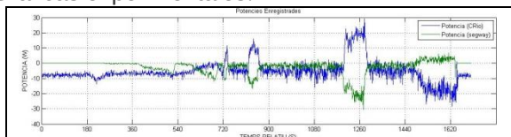
Fig.4: Prueba N°1: Desplazamiento en modo tractor.
