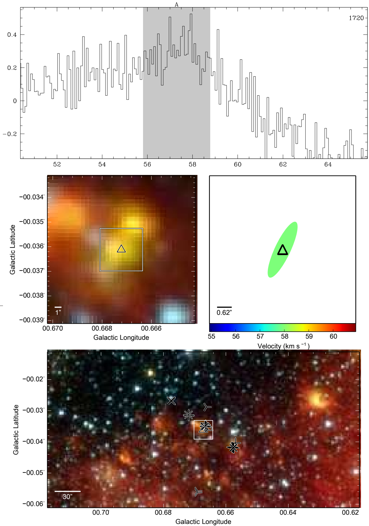
Fig. 5.— G000.667-0.036 – SF
