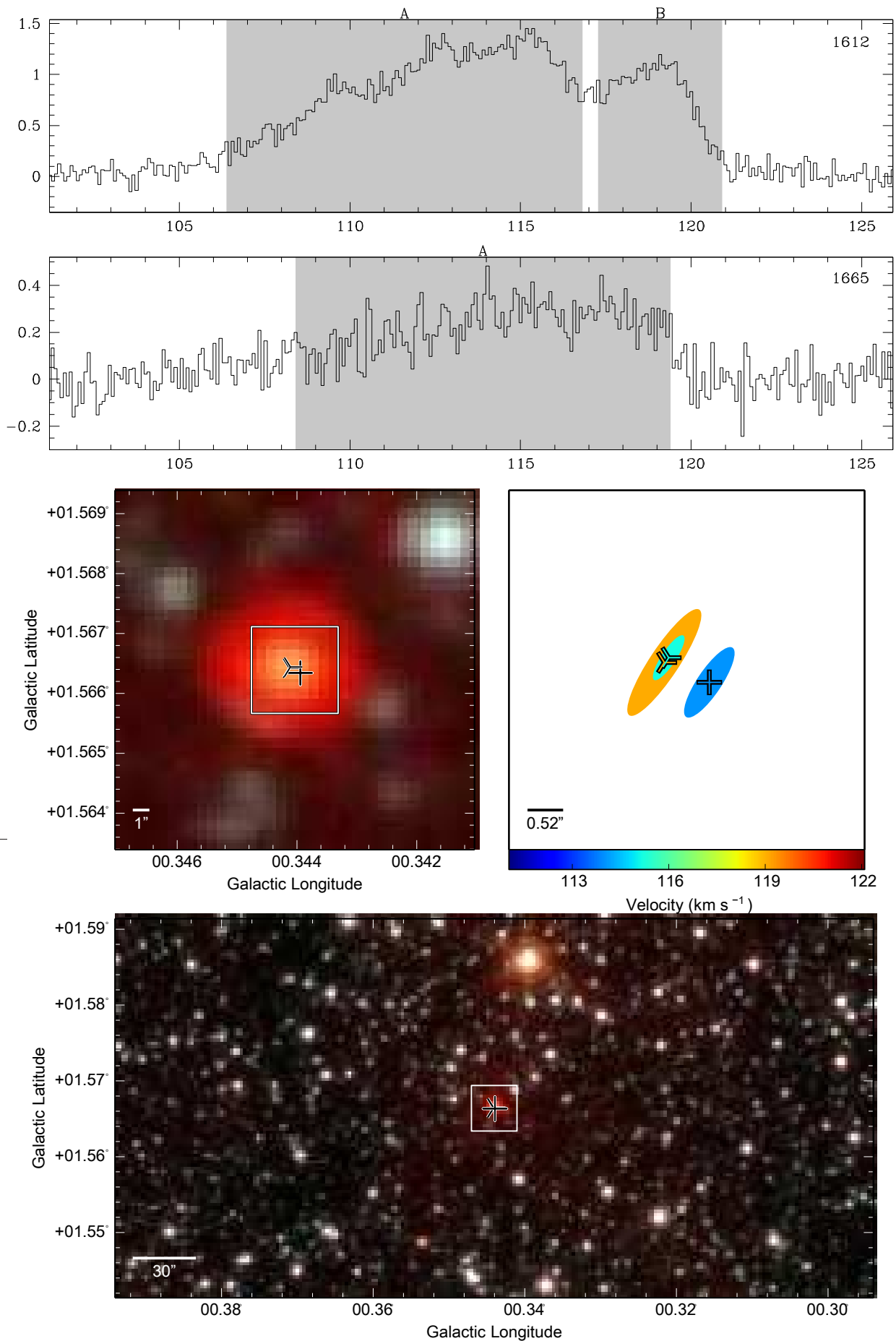
Fig. 4.— G00.344+1.566 – PN
