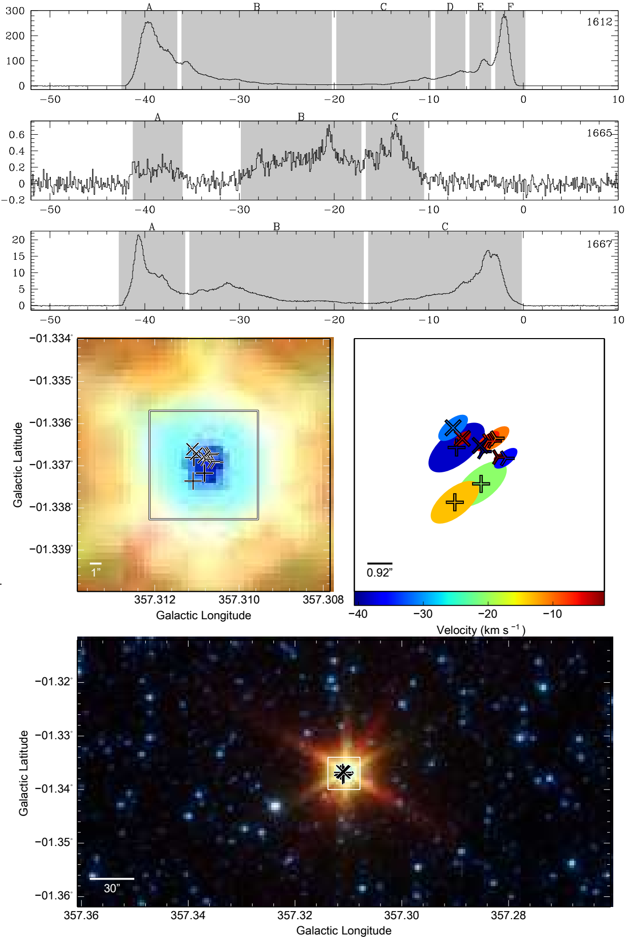
Fig. 3.— G357.311–1.337 – ES
