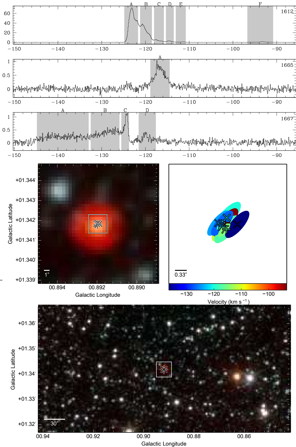
Fig. 6.— G000.892+1.342 – PN
