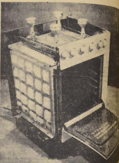
La foto muestra una cocina Ferrilloza antes de terminarse de armarse, donde se aprecian su terminación y su aislamiento total del horno con lana de vidrio.
