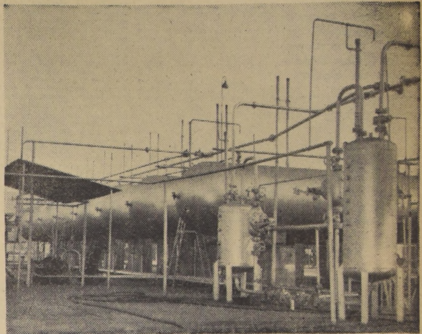
La Planta de Almacenamiento de GASCO, para gas licuado, la primera en entrar en funcionamiento. Su capacidad alcanza a las 90 toneladas y será ampliada al doble
