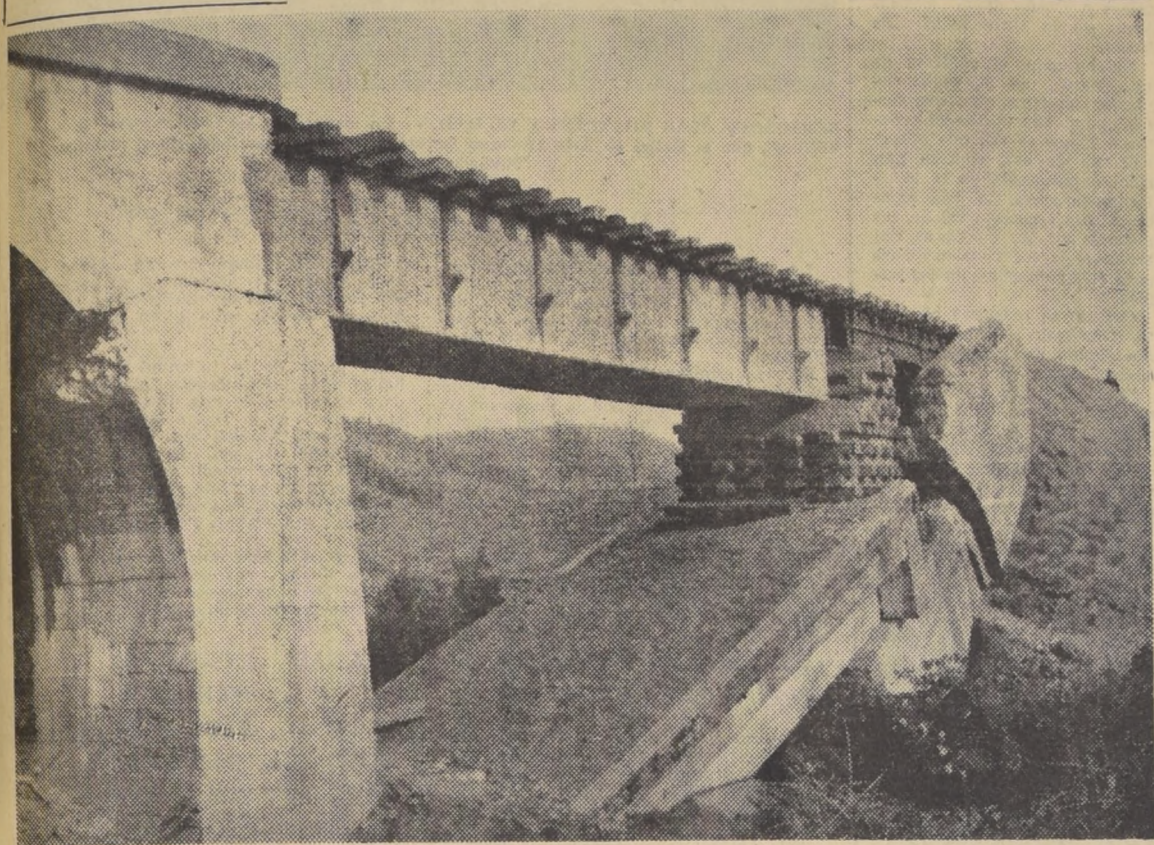
En el ramal de Loncoche a Villarrica, cerca de la Estación de Nancul, se quebraron los arcos del puente sobre el río de este nombre. Como lo muestra el grabado, de Víctor Rojas, se rompió uno de los tramos y la plataforma de cemento. Cuadrillas de obreros, sin embargo, los colocaron durmientes y otros soportes, y luego de otras reparaciones menores se estará en condiciones de restablecer el tránsito ferroviario hacia aquel balneario del Sur, que ya se hace con algunas precauciones. (Gentileza de la Empresa de los FF.CC. del Estado.)
