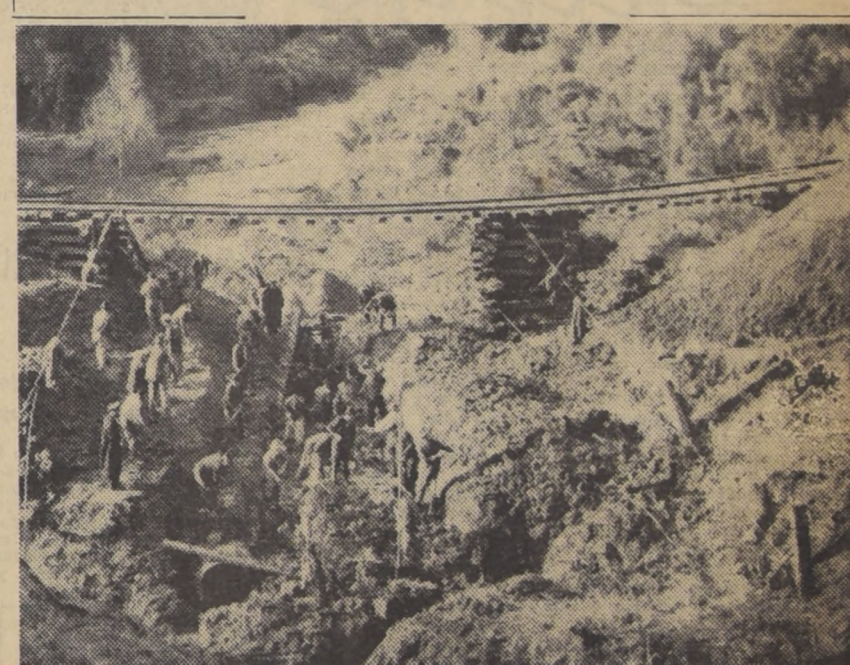
ESTO FUE UN TERRAPLEN DE unos treinta metros de largo por quince de alto, en el kilómetro 857,700 del ferrocarril longitudinal, cerca de la Estación de Lipingue. El movimiento sísmico del 22 de mayo arrastró el material pétreo hacia el río Lipingue, y la red quedó prácticamente en el aire. Semipuntalado y sujeto por cables, sin embargo, permite el paso de motocicletas, autocarritos, etc., hacia Osorno. Cincuenta obreros trabajan jornadas de nueve horas diarias para reponer cuanto antes el tránsito ferroviario hacia el sur.— (Foto de Víctor Rojas. Gentileza de la Empresa de los Ferrocarriles del Estado.)
