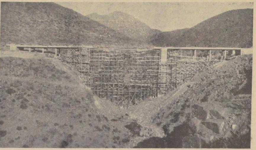
LA SERENA.— Vista panorámica del gran puente de Juan Soldado, que se construye a 32 kilómetros de La Serena. Tendrá la particularidad de cimentarse sobre un solo arco central con pilares adicionales sobre él y a sus lados. La palicera que muestra el grabado da una idea de la exuberancia del empleo de las maderas en moldes y andamios. (Fotos Raúl Salfate, Muñoz Leiva, corresponsal).
