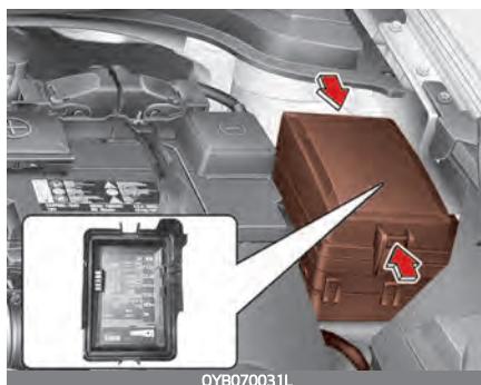
Scatola fusibili vano motore (Smartstream G1.0 T-GDi PTC solo riscaldatore)
