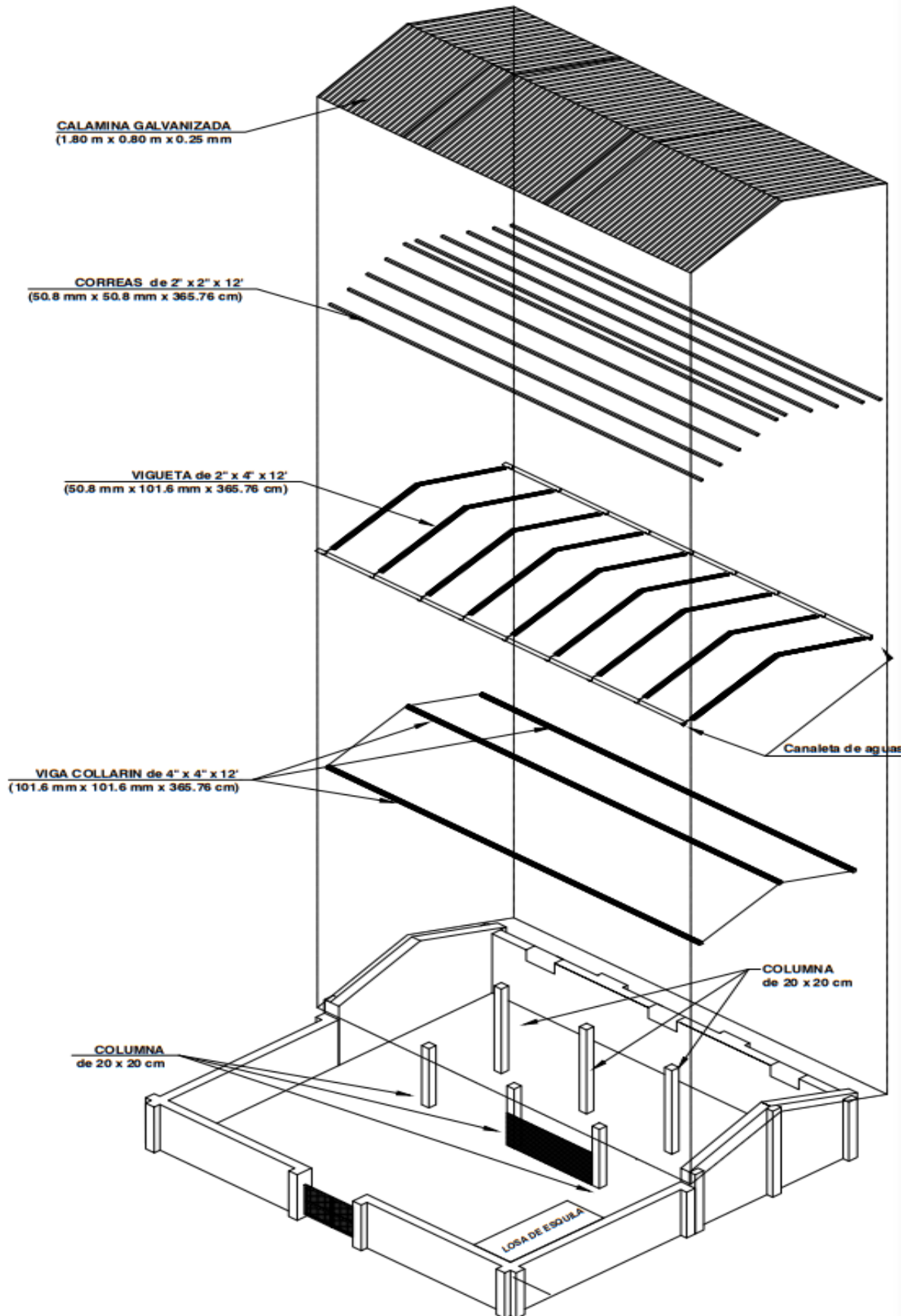
Figura 2. Isométrico de cobertizo con estructura de soporte de techo con tijerales de madera aserrada para módulos para el resguardo de ganado (cobertizos)
