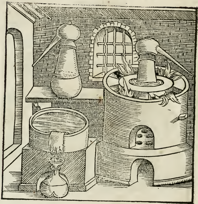
De Furno descensorio. Caput V.
