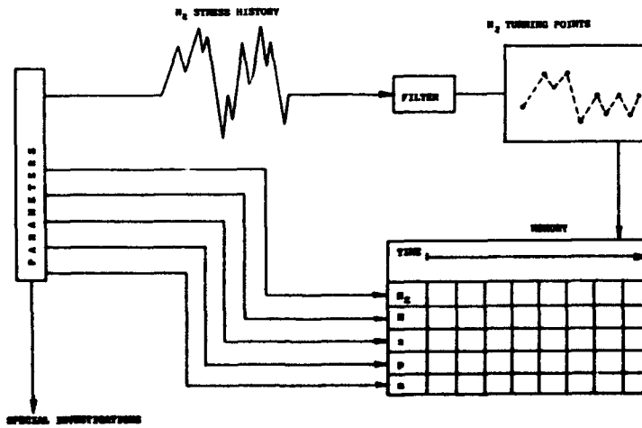
Fig.3: Parameters Process
