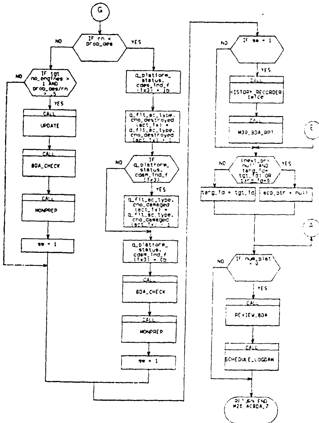
Subroutine M26_AC8DA_2 (d)
