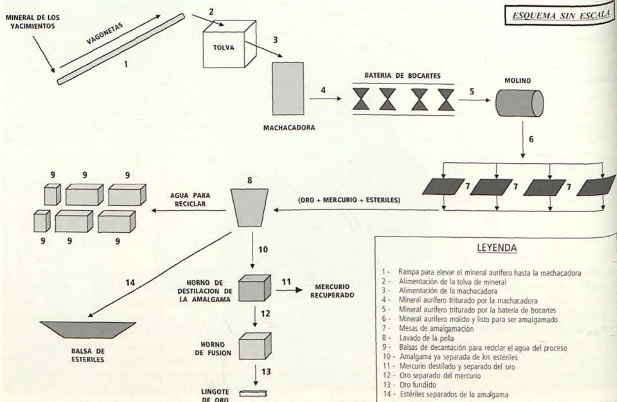
Figura 4. Esquema simplificado del funcionamiento de la instalación metalúrgica aurífera por amalgamación de la empresa Explotaciones y Minas Auríferas de Rodalquilar S.A. (año 1929).
