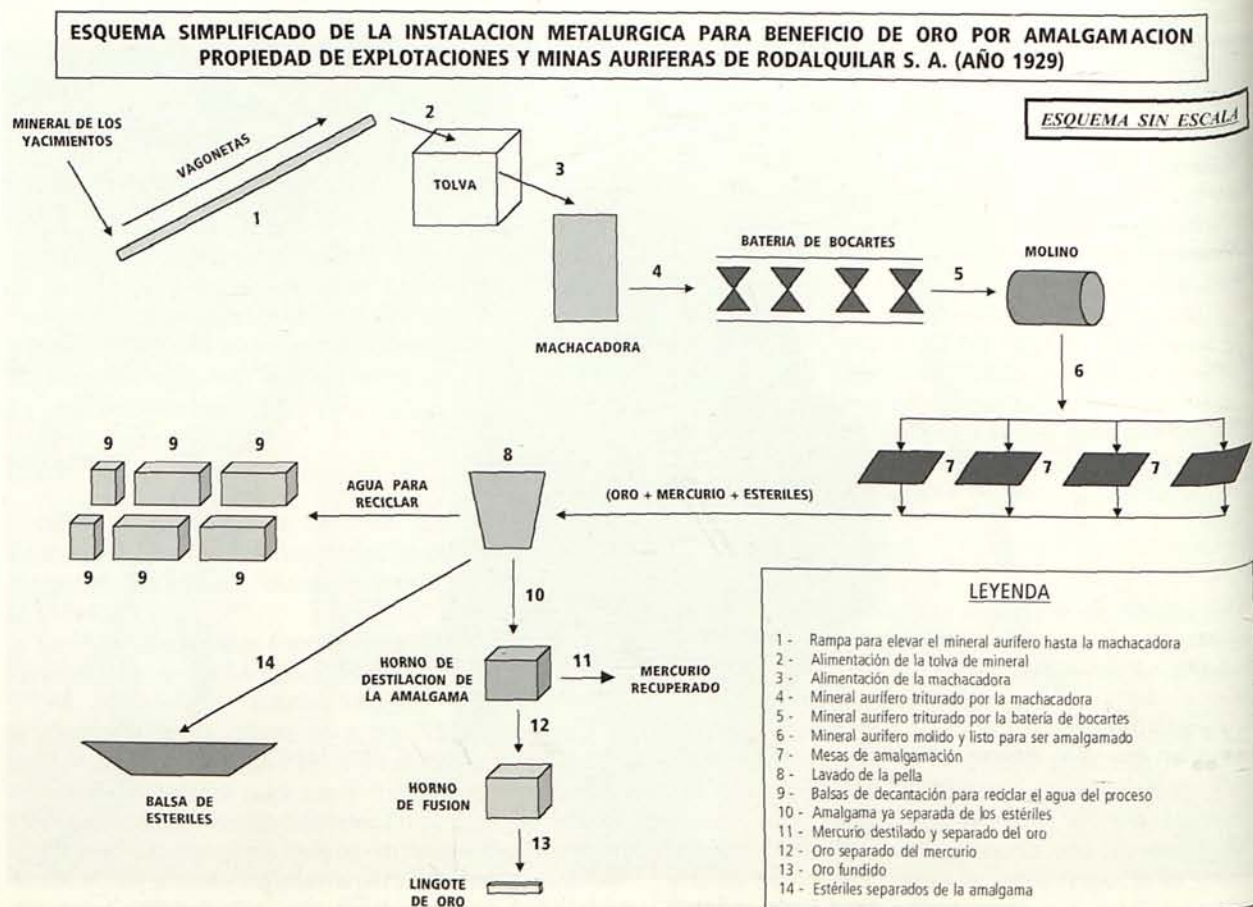
Figura 4. Esquema simplificado del funcionamiento de la instalación metalúrgica aurífera por amalgamación de la empresa Explotaciones y Minas Auríferas de Rodalquilar S.A. (año 1929).
