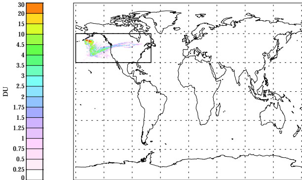
Okmok 12-20 Jul 2008
