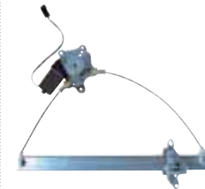
NSU8-B680EL NSU8-B680ER U13/ 风神 FR WINDOW REGULATOR W/MOTOR 80721-1E700 FL 80720-1E700 FR
