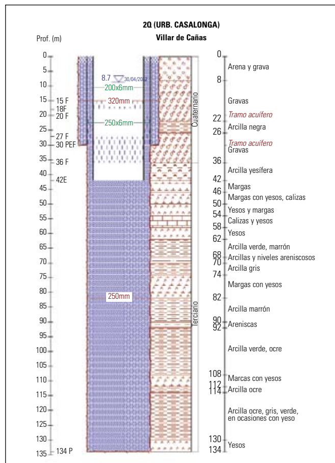
Figura 6.2. Perfil litológico del sondeo 2Q (Martínez, 2002b).
