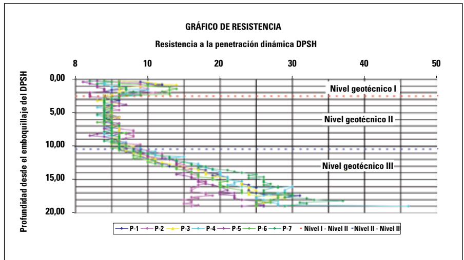
Figura 5. Evolución del golpeo DPSH en función de la profundidad.
