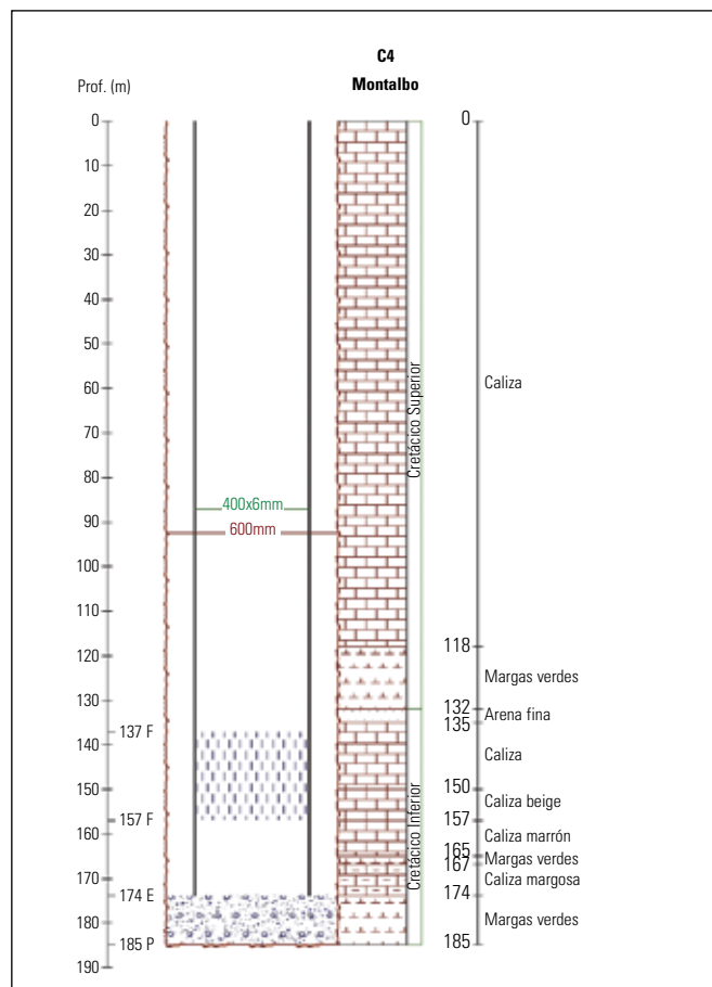
Figura 5.2. Perfil litológico del sondeo C4 (Martínez, 2006b).
