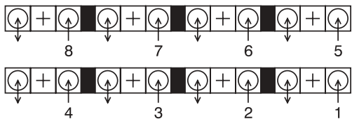
Etiqueta de compartimento de entradas
