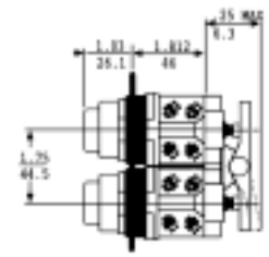
Botones entrelazados mecánicamente
