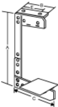
Colgador universal
