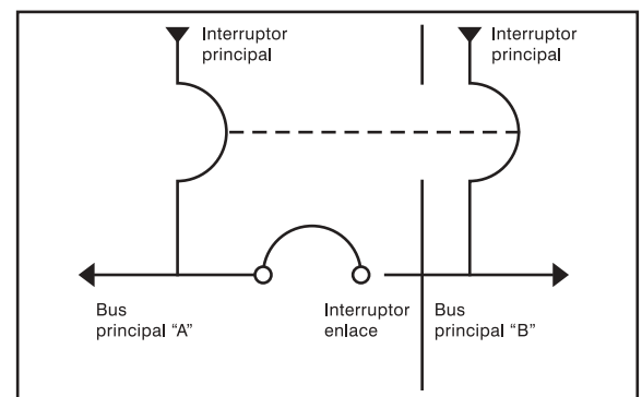
Sección principal-enlace/sección principal
