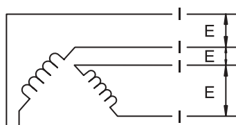
2 fases - 4 hilos
