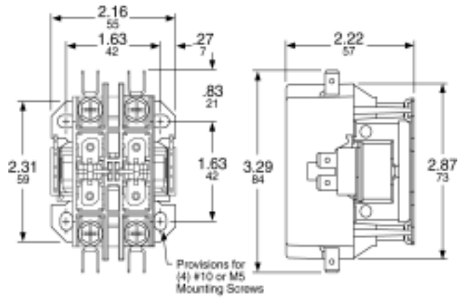
Tipo DP - 2 polos 20 a 40 A a plena carga.
