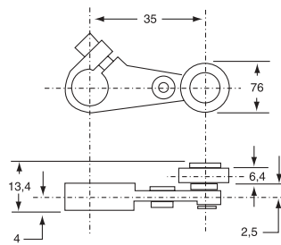
Brazo estándar
