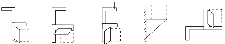
Nivelado con el techo en zeta, abertura lateral
