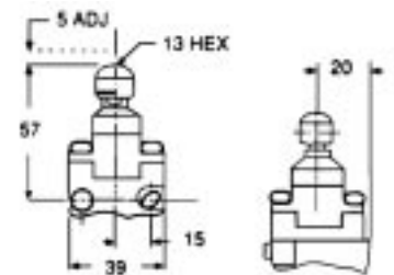
Cabeza pulsadora ajustable
