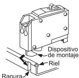
QOGFI 2 polos
