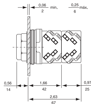
No iluminado KR4, KR5
