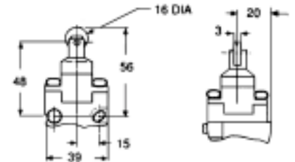
Pulsador con roldana
