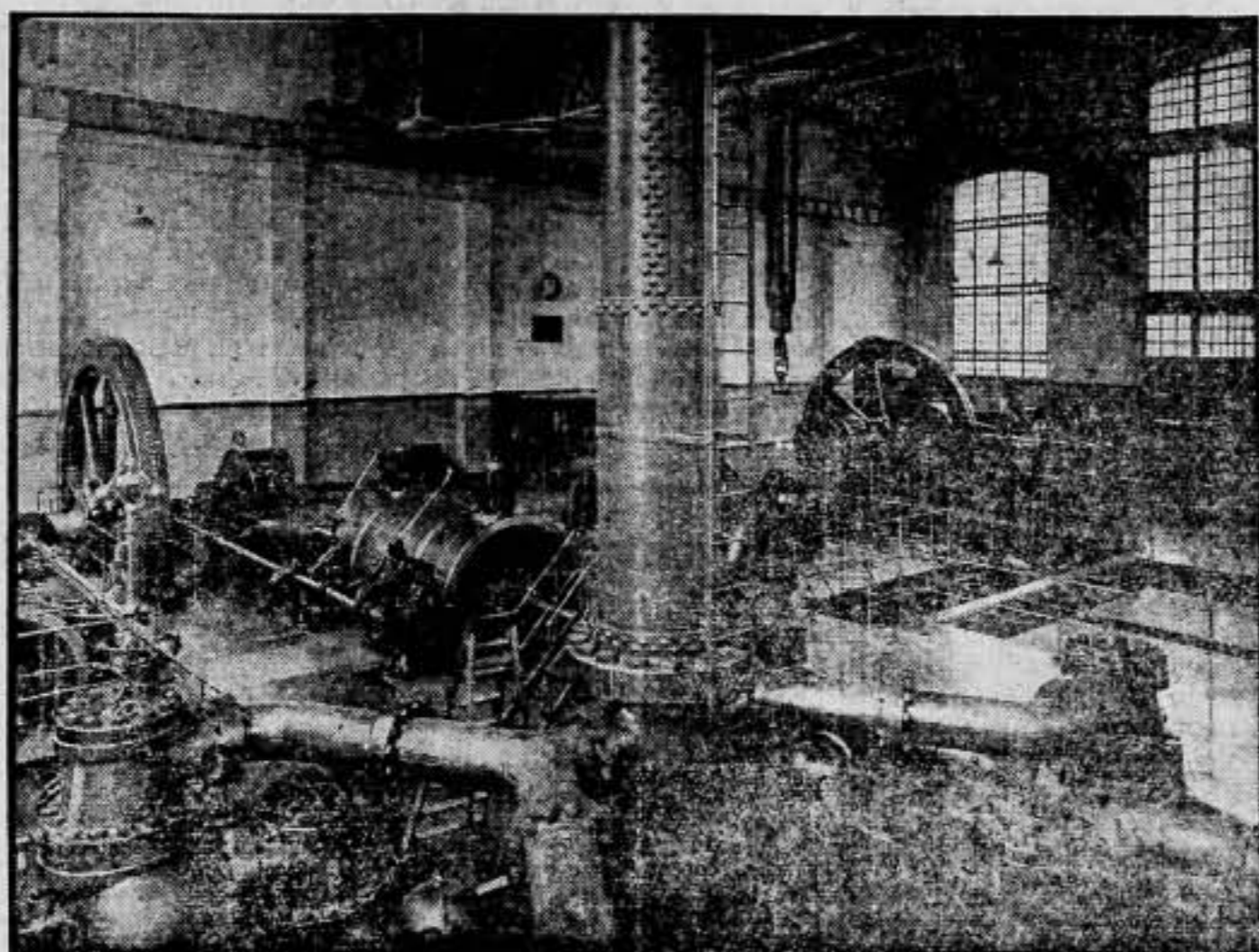
SALA DE MAQUINAS CENTRAL CORNELLA
