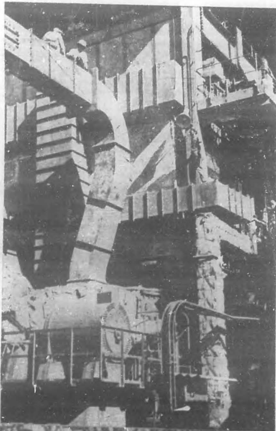
Aspecto de una de las tres calderas de 100,000 libras cada una que se instalan en el central Guiteras.
