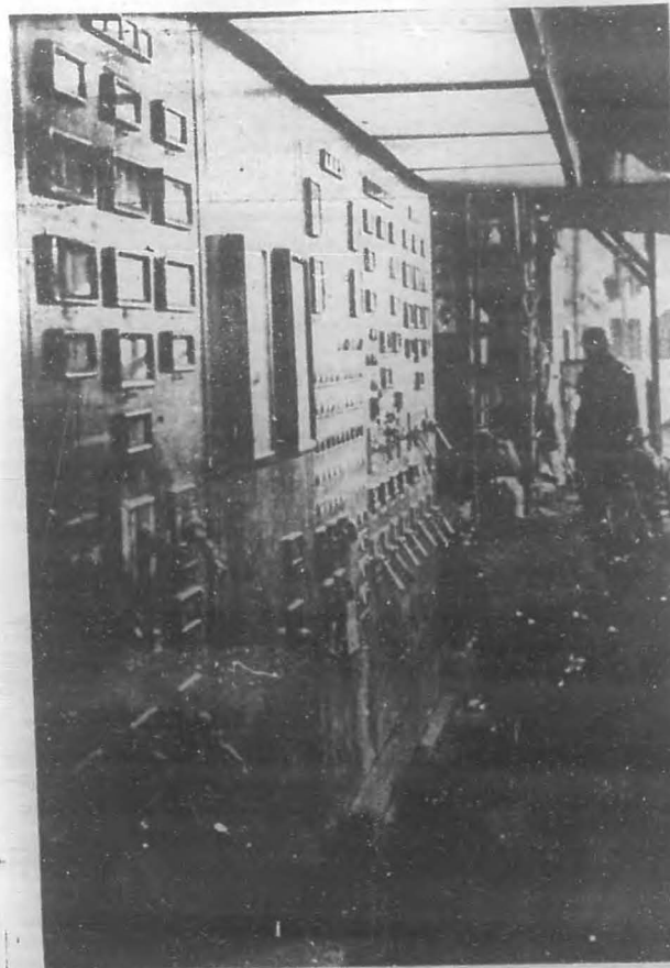
Pizarra de control de la planta termoeléctrica que se instala en el central Antonio Guiteras.
