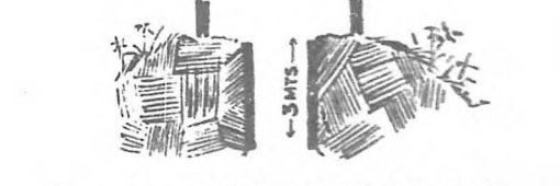
El pozo debe estar forrado por una pared interior de tres metros de profundidad por lo menos. Esa pared debe tener un repello que impida la filtración.
