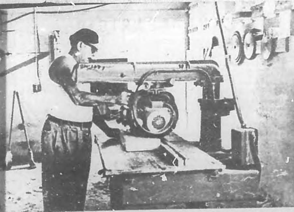
Primero los tabloncillos se convierten en pequeños bloques y después se cortan las tabillas, de cada una de las cuales salen siete lápices.
