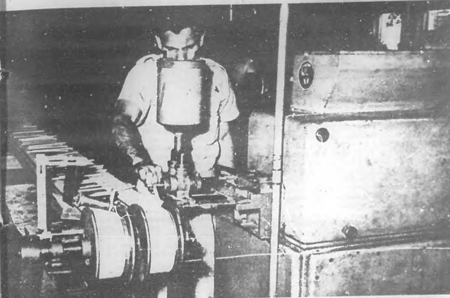
En este aparato los lápices reciben la primera mano de pintura y se secan en la estera durante su breve recorrido hasta el depósito.
