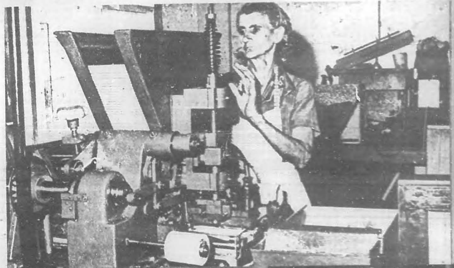
En este aparato los lápices reciben la primera mano de pintura y se secan en la estera durante su breve recorrido hasta el depósito.
