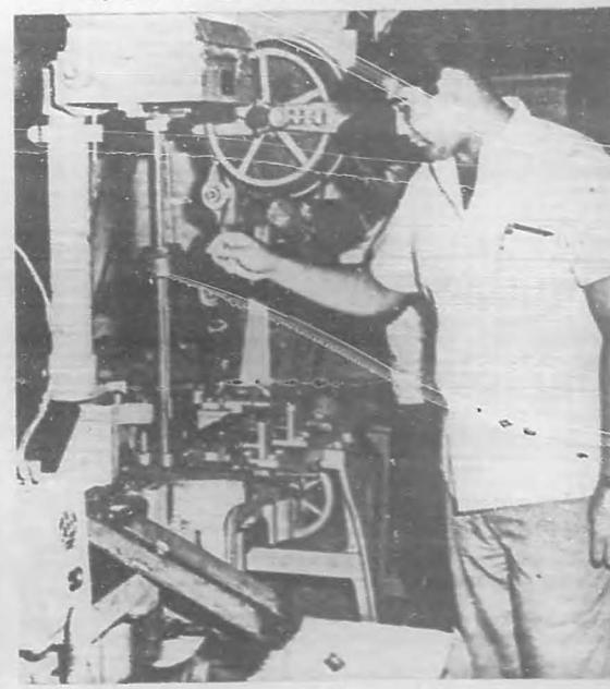
Un "close-up" de la máquina "Johnson", que fue adaptada por el obrero Gustavo García, la cual está produciendo 80,000 tapas encorchadas en cada turno de ocho horas, (240,000 en tres turnos). El inspector Arturo Reyes, está chequeando la calidad de la producción.
