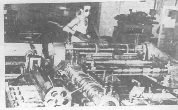
Cuchilla "duplex", automática. Corta cuerpos de "411" de altura, con una producción de 5,000 láminas o planchas, cada 8 horas, (15,000 en los tres turnos.) Las planchas son de procedencia soviética o japonesa.
