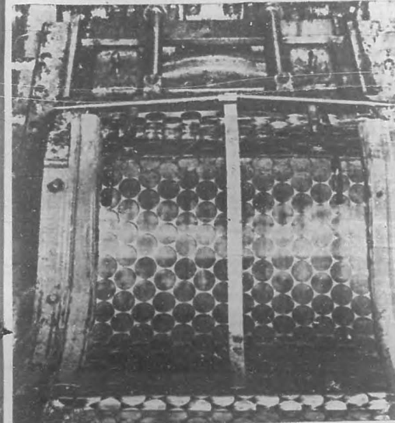
Esta máquina formidable desarrolla una presión fantástica de cuarenta toneladas, sobre las planchas litografiadas con los nombres de las cervezas o refrescos. Cada lámina produce 352 tapas corona, con una producción total de 54,000 gruesas en los tres turnos de ocho horas cada turno, con un promedio de un millón seiscientos veinte mil mensuales.
