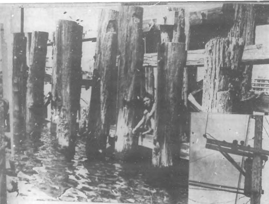
18—Pilotes de un muelle. Esos troncos, preferentemente de ácana, guayacán y jiquí, son incorruptibles y se mantienen intactos debajo del agua durante siglos.
