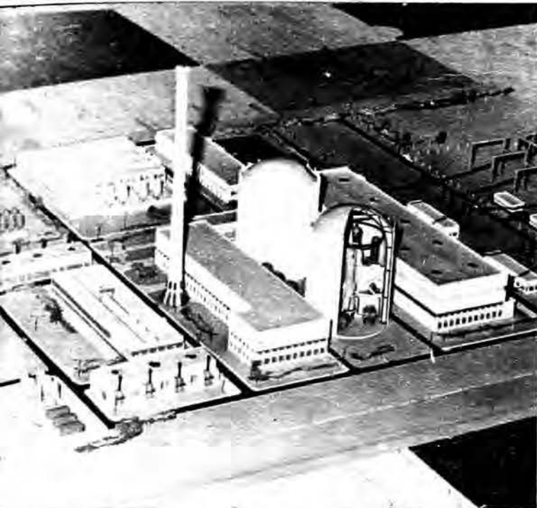
Maqueta de la planta electrónuclear 800 MW en su primera fase.
