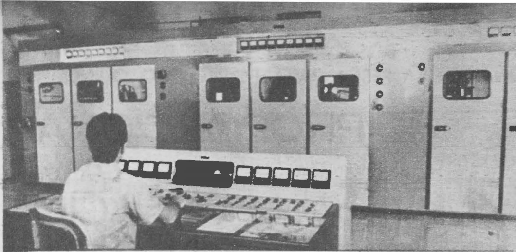
Equipo transmisor de 150 Kw, uno de los dos más potentes de Cuba.
