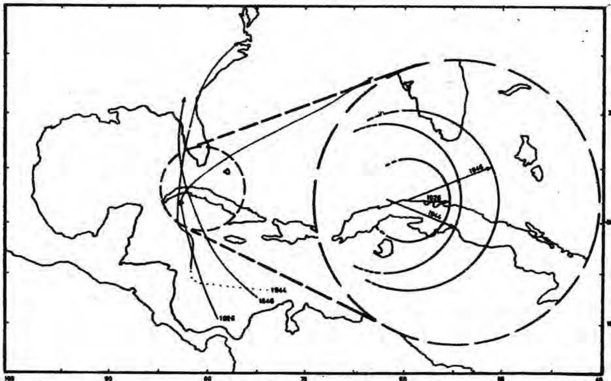
Trayectorias de los huracanes de 1846, 1926 y 1944 y áreas aproximadas de los vientos huracanados sobre Cuba.
