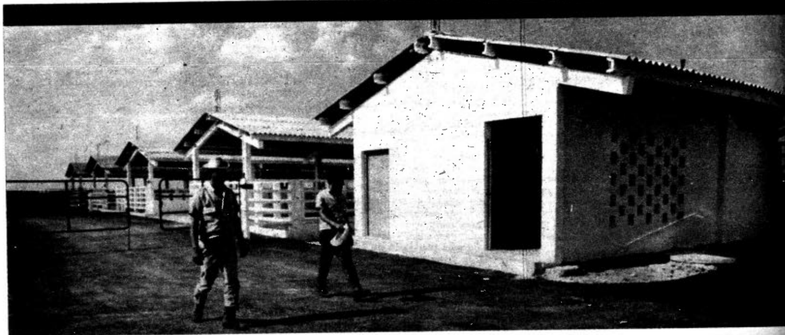
Uno de los más grandes planes de producción de la región es la granja pecuaria Dos Ríos, que proyecta construir 17 vaquerías modernas, de ordeño mecánico. He aquí a una de ellas lista para funcionar.
