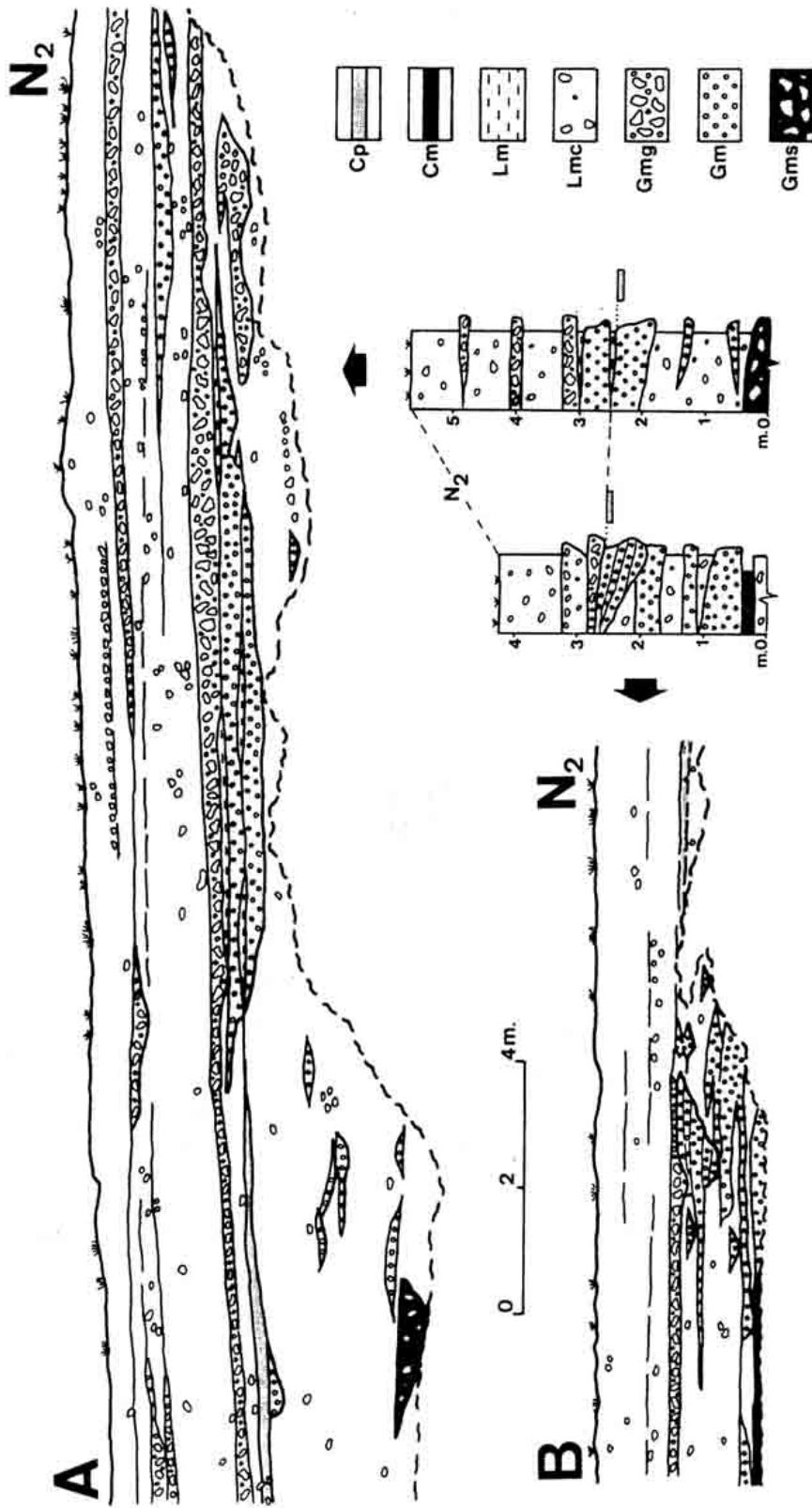
Fig. 6. Esquemas sedimentológicos y perfiles sintéticos de dos afloramientos de la unidad U 2 (localización en Figura 2). Sedimentological sketches and synthetic profiles of two outcrops of the U 2 unit (location in Figure 2).
