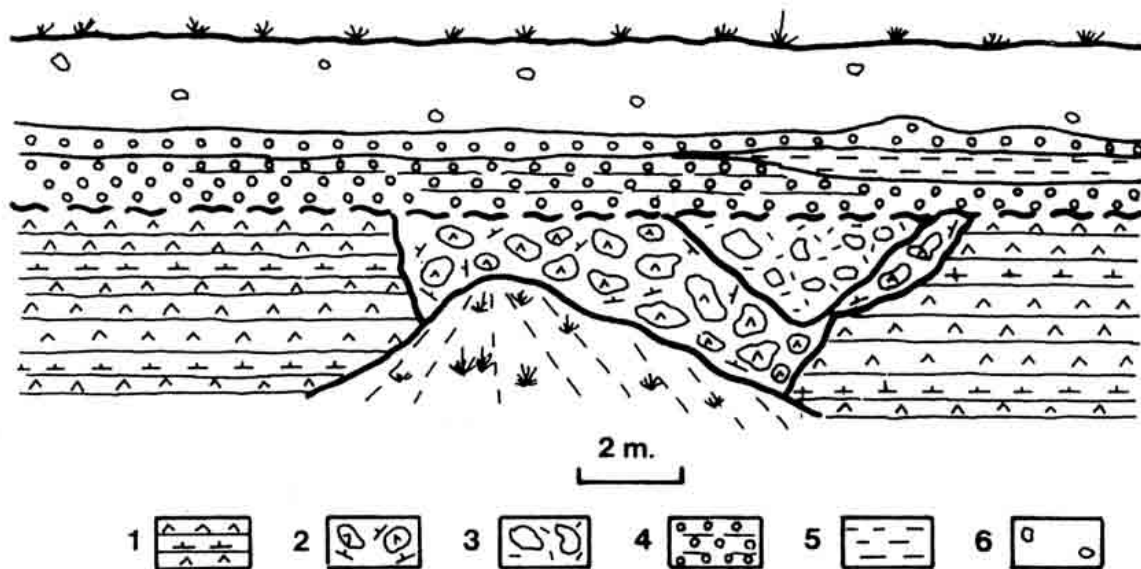
Fig. 5. Relleno de paleodolina en embudo correspondiente a la unidad U 3 . Esta paleodolina está truncada y fosilizada por el depósito sin cementar de la unidad U 2 . 1: Sustrato yesífero con intercalaciones margosas. 2: Bloques de yeso empastados en material margoso. 3: Masa caótica cementada de bloques empastados en una matriz de limo yesífero. 4: Facies Gm. 5: Facies Lm. 6: Facies Lmc.
