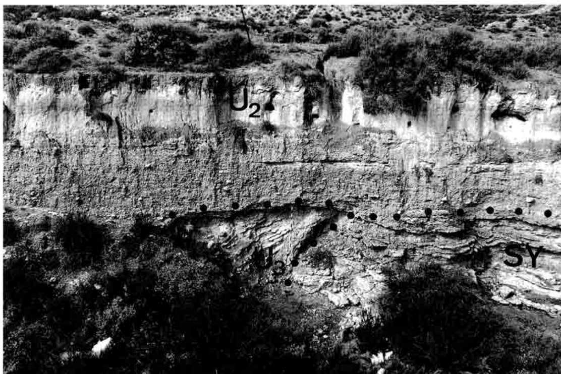
Foto 2. Depósito de la unidad U 2 que se superpone al depósito de la unidad U 3 y al sustrato mioceno (SY), en discordancia angular y en disconformidad respectivamente.
