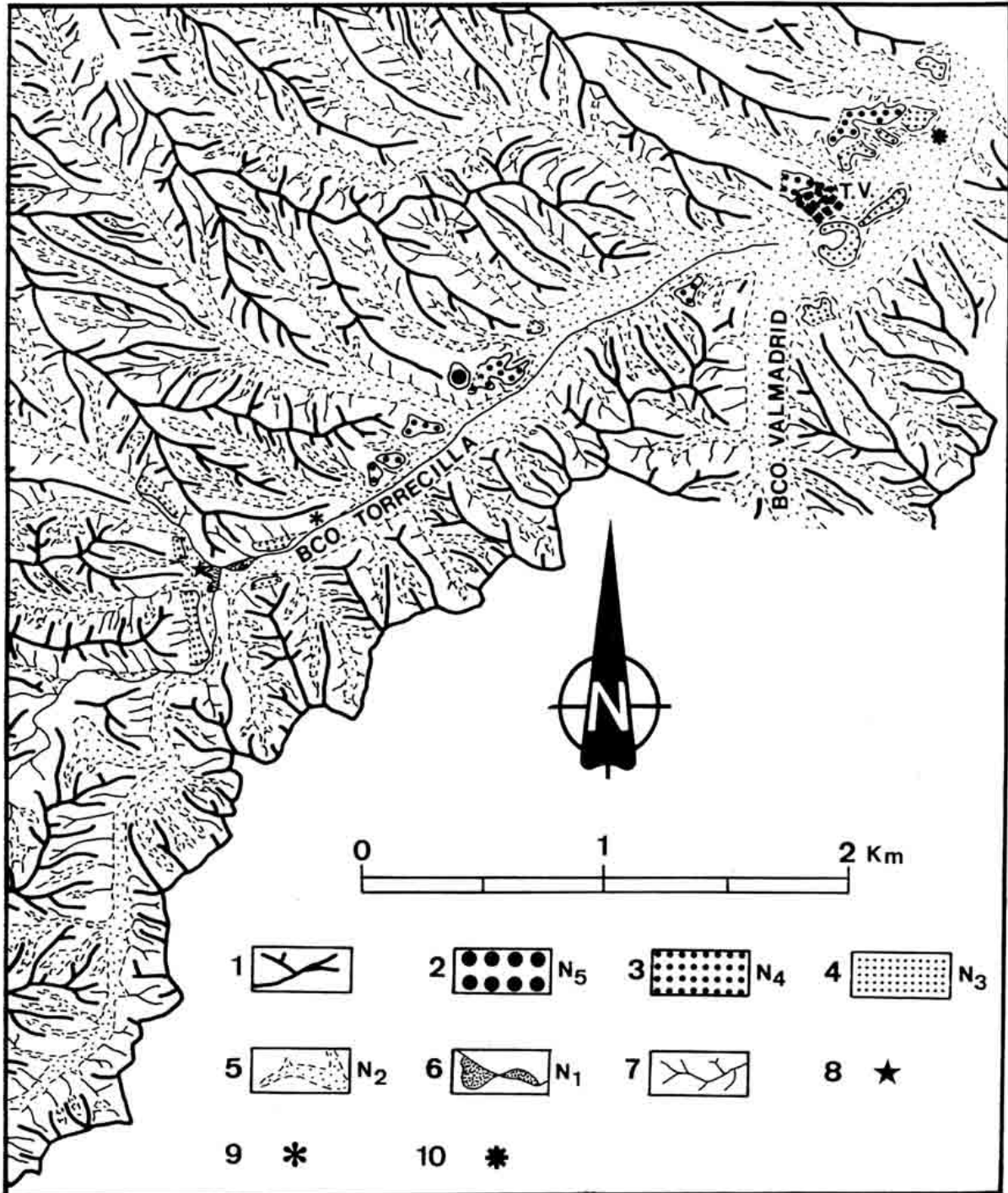
Fig. 2. Mapa geomorfológico del Barranco de Torrecilla. 1: Interfluvios en materiales yesíferos. 2: Nivel N 5 . 3: N 4 . 4: N 3 . 5: N 2 . 6: N 1 . 7: Incisiones lineales. 8: Situación de los esquemas de la Figura 6. 9: Situación del Perfil 1 de la Figura 4. 10: Situación del Perfil 2 de la Figura 4. T. V.: Torrecilla de Valmadrid. Geomorphologic map of the Torrecilla Arroyo. 1: Divides in gypsiferous materials. 2: Level N 5 . 3: N 4 . 4: N 3 . 5: N 2 . 6: N 1 . 7: Linear incision. 8: Situation of the sketches in the Figure 6. 9: Situation of the Profile 1 in the Figure 4. 10: Situation of the Profile 2 in the Figure 4. T. V.: Torrecilla de Valmadrid.
