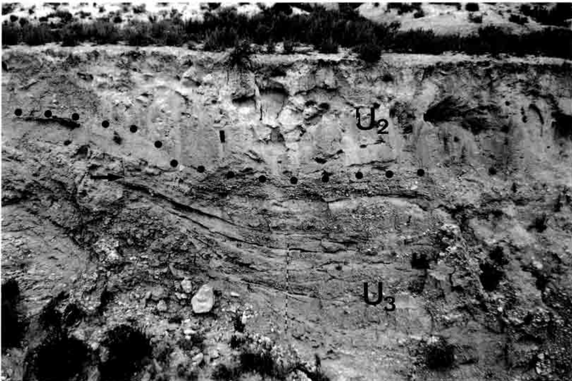
Foto 1. Abanico de capas en el depósito de la unidad U 3 , correspondiente al margen de aguas arriba de un foco subsidente. Este abanico de capas se apoya sobre un residuo kárstico con un dispositivo en onlap . El depósito de la unidad U 2 se superpone al de la unidad U 3 . La flecha señala una diaclasa que se interrumpe en el contacto entre ambas unidades.
