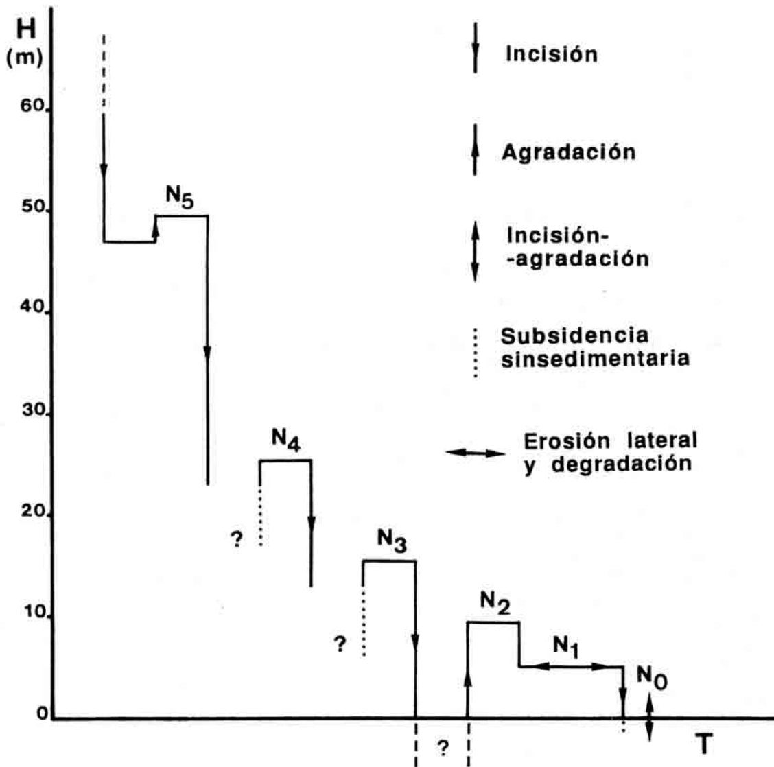
Figura 7. Evolución del Sistema Morfo-Sedimentario. H: Altura respecto del thalweg o del nivel de base en cada sector. T: Tiempo (sin escala). Evolution of the Morpho-Sedimentary System. H: Height in respect to the thalweg or to the base level for each sector. T: Time (no scale).
