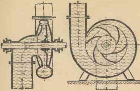
8. Niskopiętna pompa odśrodkowa.
