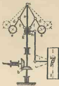
Regulatur Watta.
