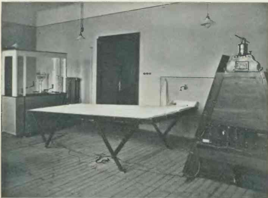
7. Aparat do badania szoferów i motorniczych tramwajowych. Badany stojąc na zwykłym stole np. motorowego tramw., ma zupełnie wrażenie jakby jechał, gdyż film przesuwają przed nim na płótnie obraz ulicy z wozami, autami, przechodniami, stacjami, zwrotnicami i t. d. Z pomocą bardzo prostych ruchów korb i dzwonka badany może zmieniać szybkość swego wozu, stawać na stacjach, uważać podczas jazdy, aby nikogo nie przejechać, wymijać inne wozy i t. p. Osobne przyrządy rejestrujące zapisują wszystkie błędy badanego, czy za szybko nie jechał, czy stanął na stacji, czy nie przejechał kogo, czy wyłączył prąd na zwrotnicy i t. p. Temperament badanego ujawnia się przy tym badaniu bardzo widocznie.
