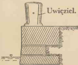
Przekrój muru bulwarowego.
