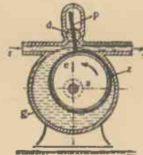
4. Pompa z tłokiem obrotowym.
