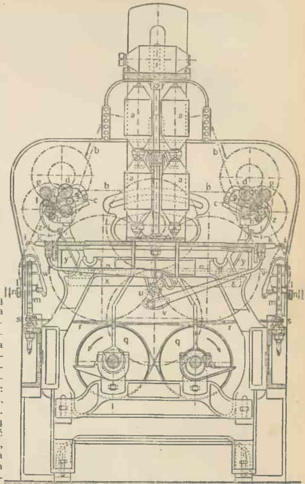
Pierścieniowa maszyna przędzalnicza.
