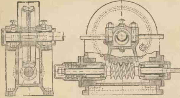
Przekładnia ślimakowa.
