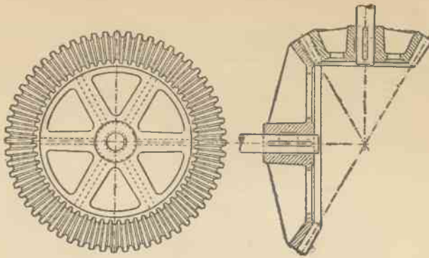
Tryby stożkowe.
