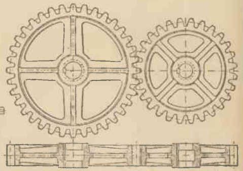
Przekładnia trybowa (tryby czołowe).
