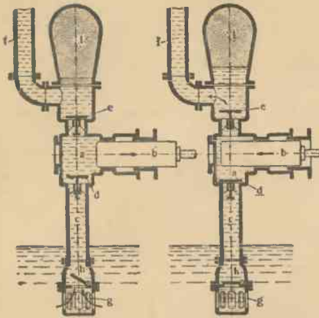
1. Prosta pompa ssąco-tłocząca.
