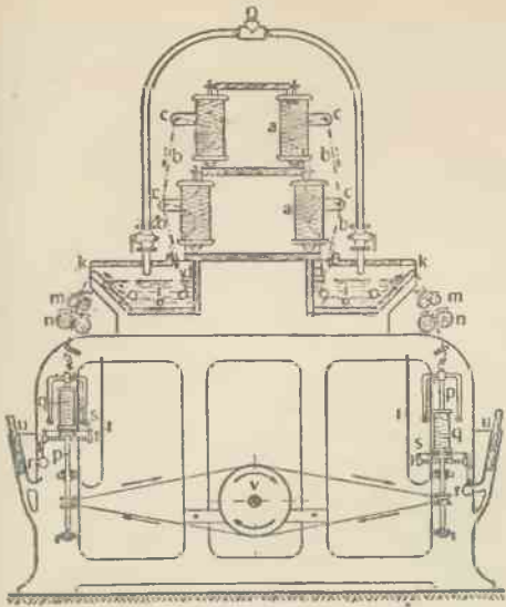
Maszyna do przędzenia lnu.
