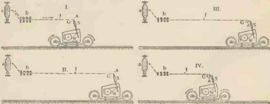
Cztery okresy pracy selfaktora.
