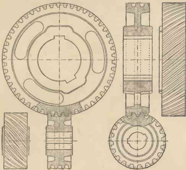
Tryby śrubowe.
