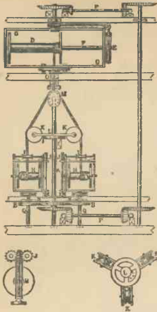
Maszyna powroźnica do kręcenia lin.
