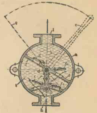
6. Podwójnie działająca pompa skrzydłowa.
