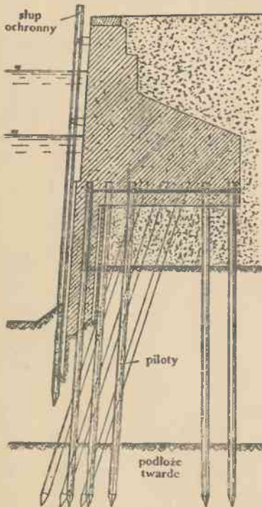
Przekrój muru bulwarowego.
