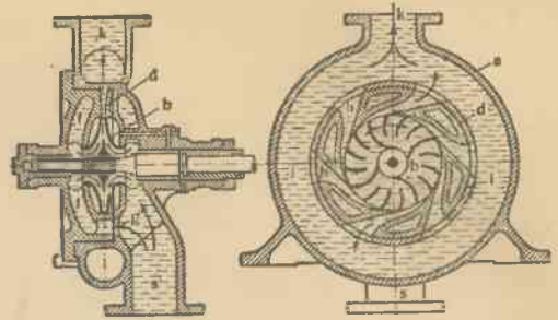
9. Wysokopiętna pompa odśrodkowa.
