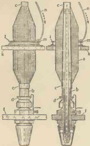
Wrzeciono maszyny pierścieniowej.
