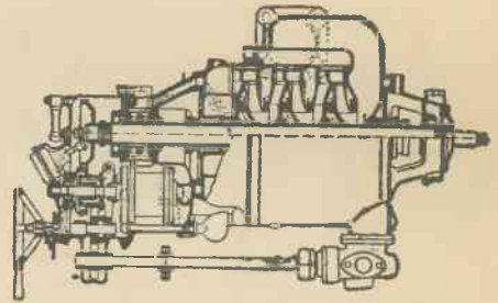
4. Pompa odśrodkowa dla sikawki.
