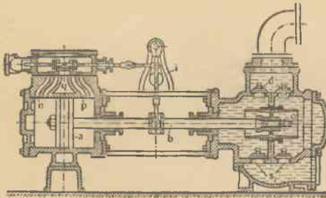
3. Pompa parowa (podwójna).
