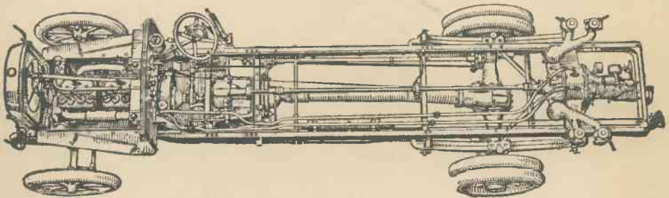
5. Podwozie samochodowe z wbudowaną pompą.
