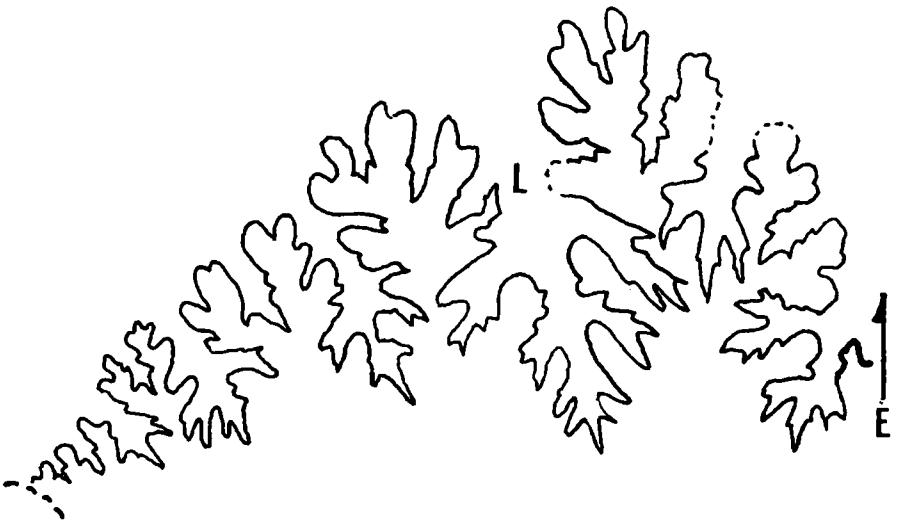
Figura 3.— S. (Strigoceras) truellei ; línea de sutura de JCe1.3.40; D = 43 mm.
